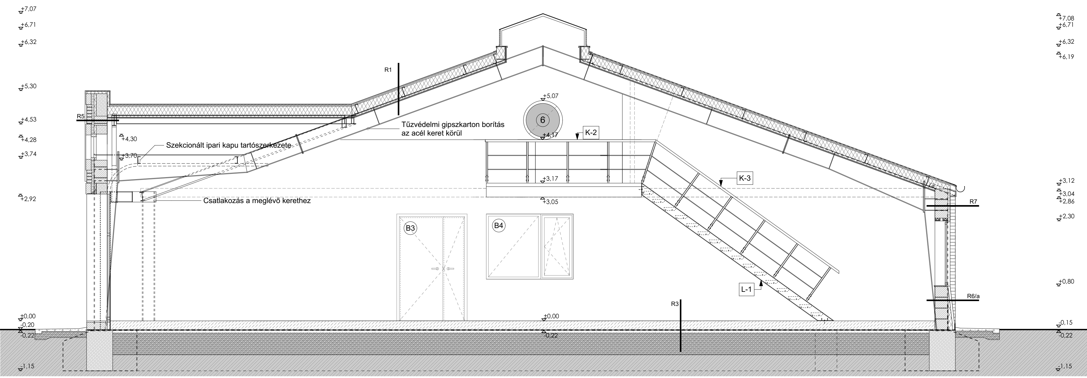
B2-B2 METSZET
