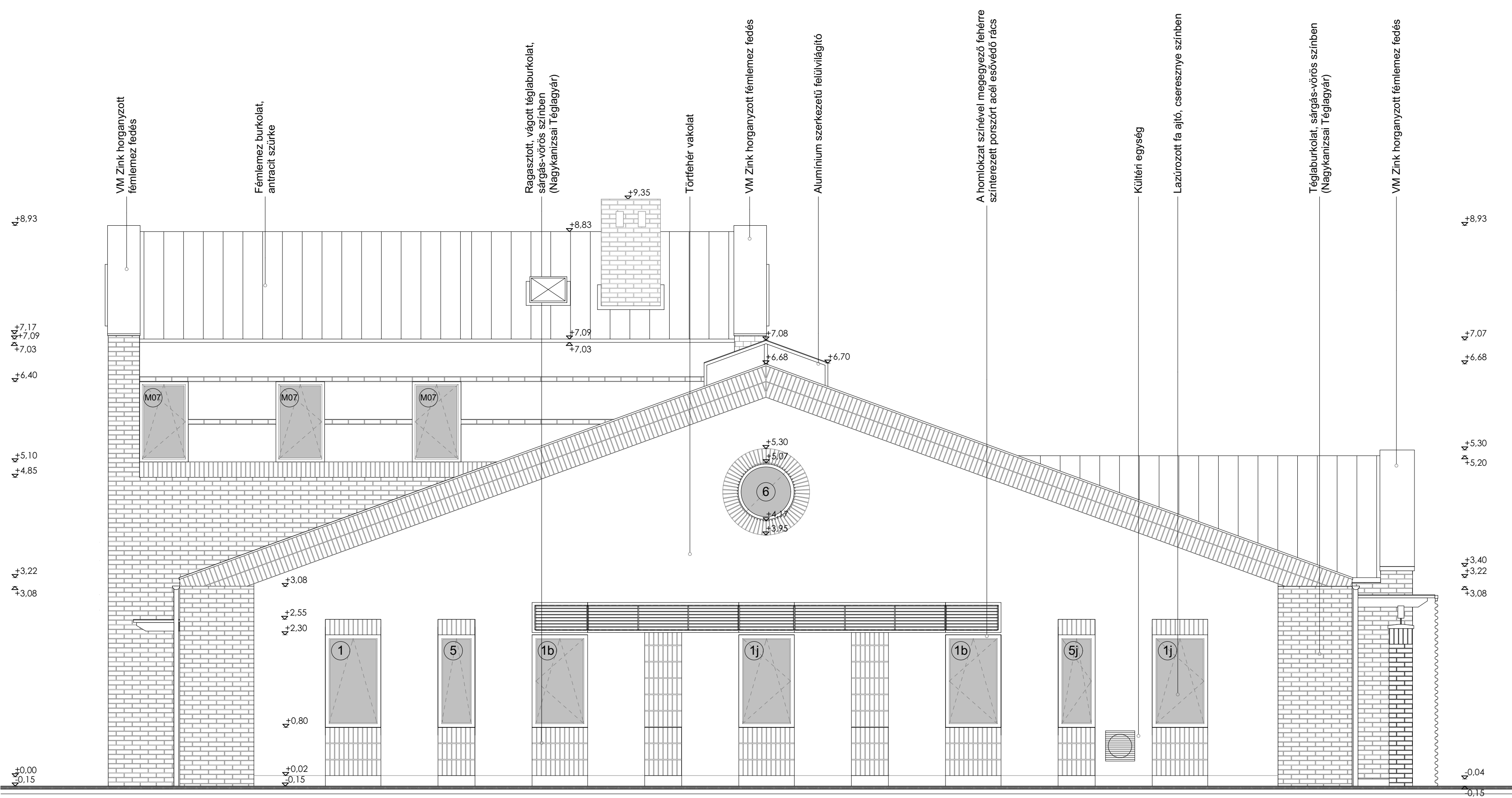
ÉSZAK-NYUGATI HOMLOKZAT
