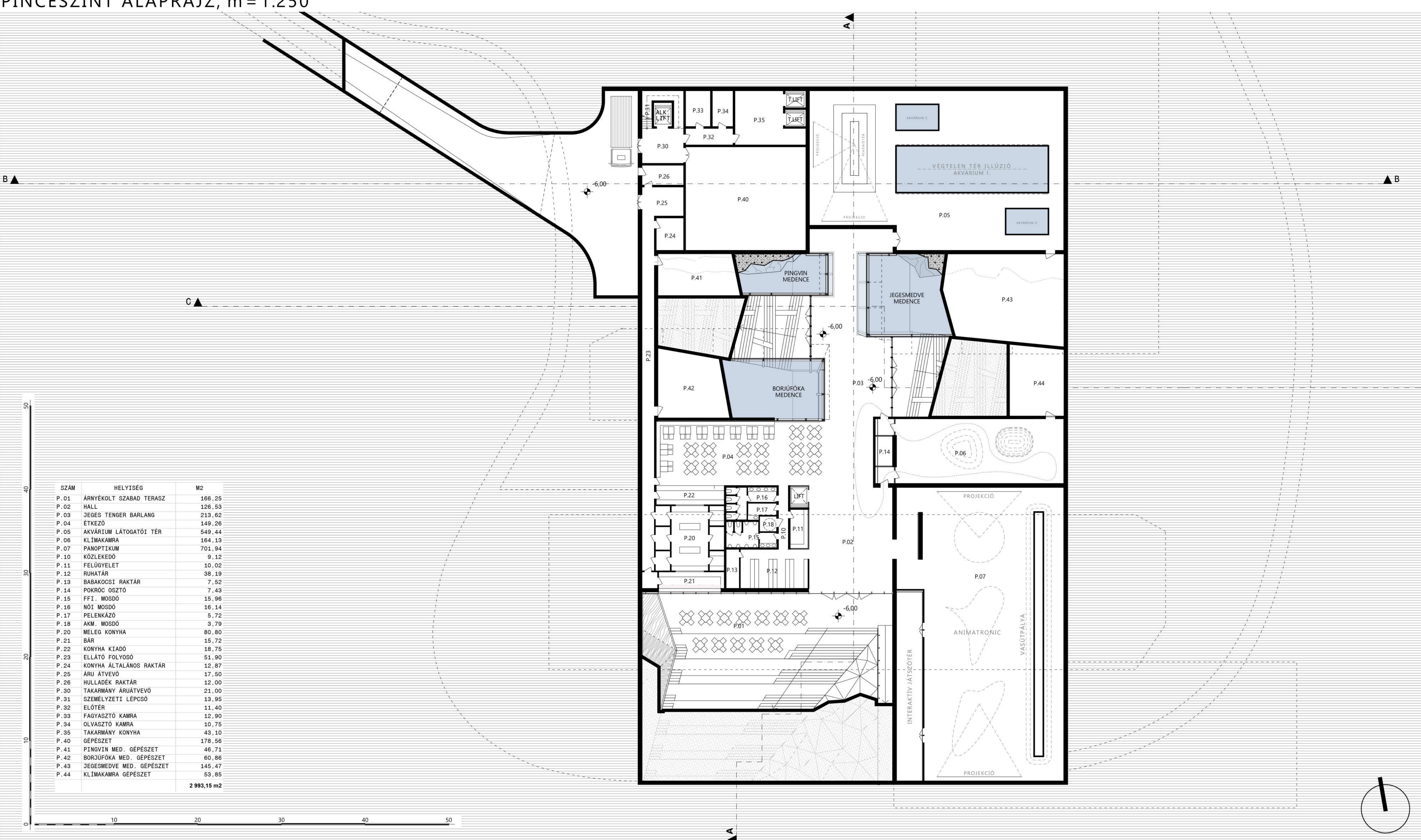
PINCESZINT ALAPRAJZ, m = 1:250
