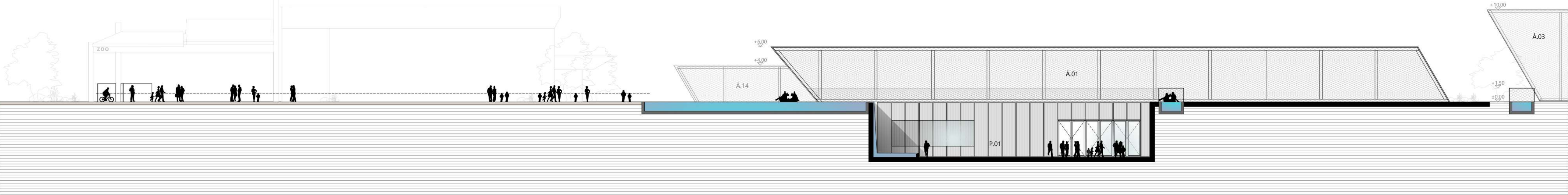
D-i HOMLOKZAT, m = 1:250
