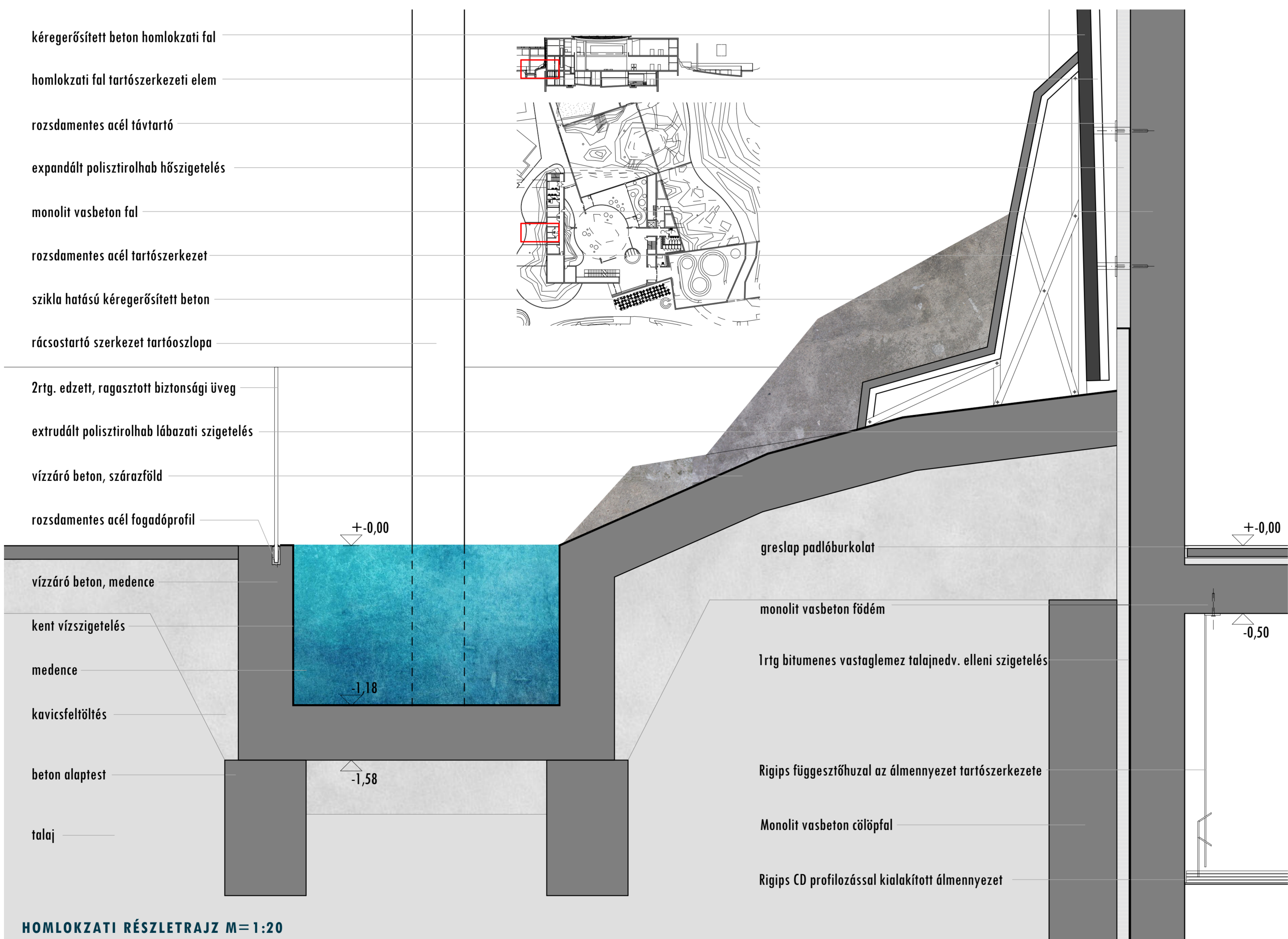
HOMLOKZATI RÉSZLETRAJZ M=1:20
