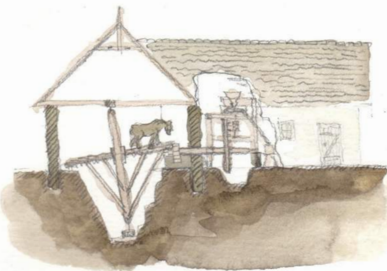
TIPRÓMALOM SZERKEZETE (ÁLLATI ERŐVEL HÁTTOTT)
