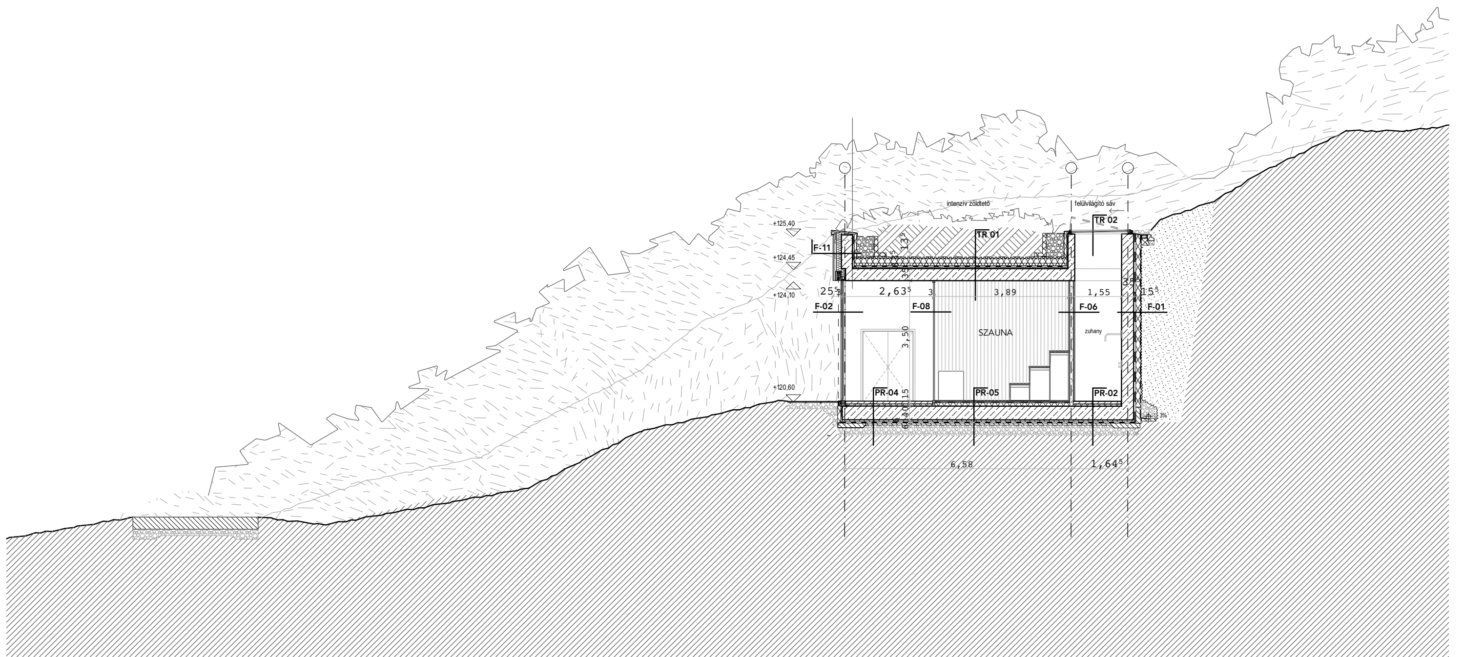
D-D KERESZTMETSZET M=1:300, M=1:100
