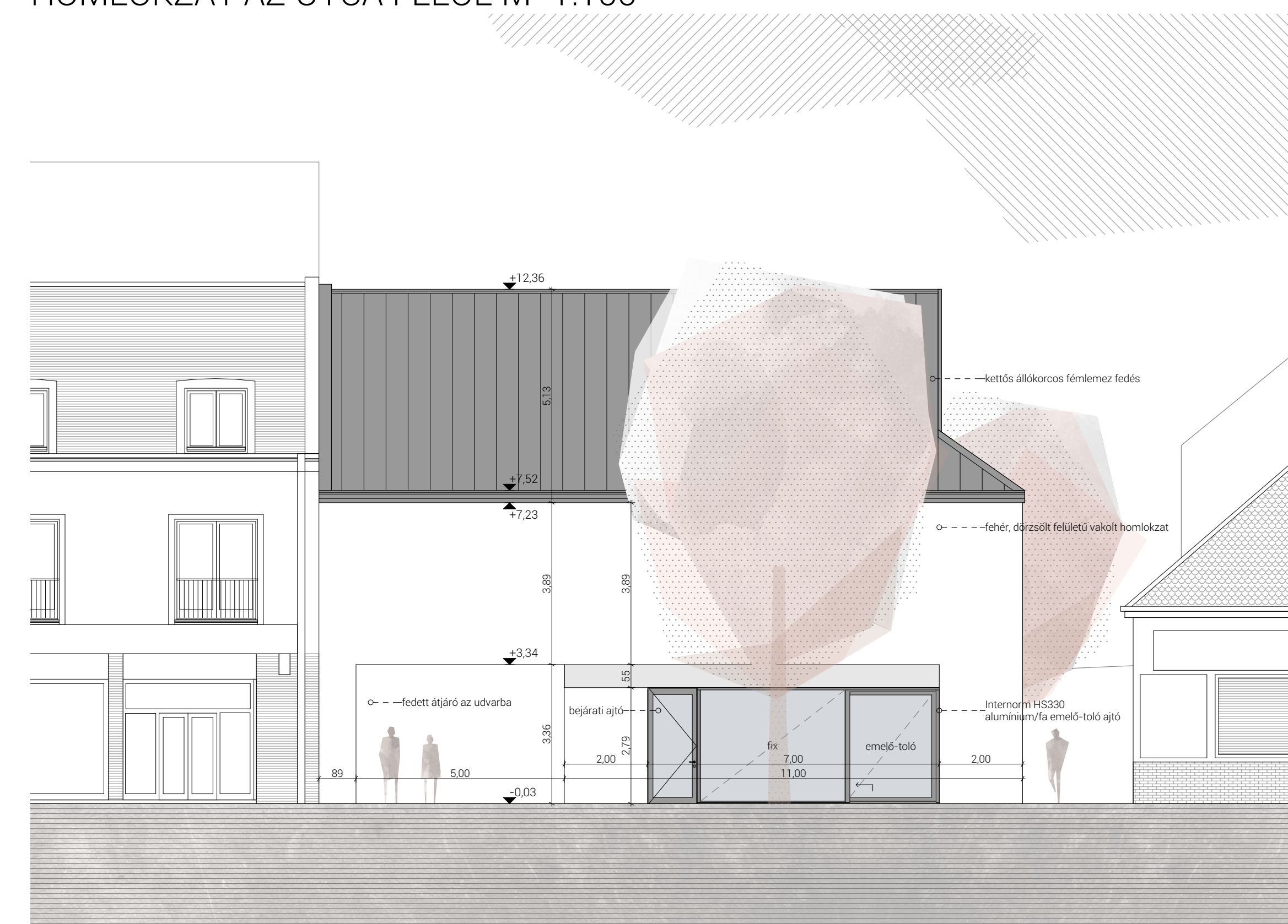
HOMLOKZAT AZ UTCA FELŐL M=1:100
