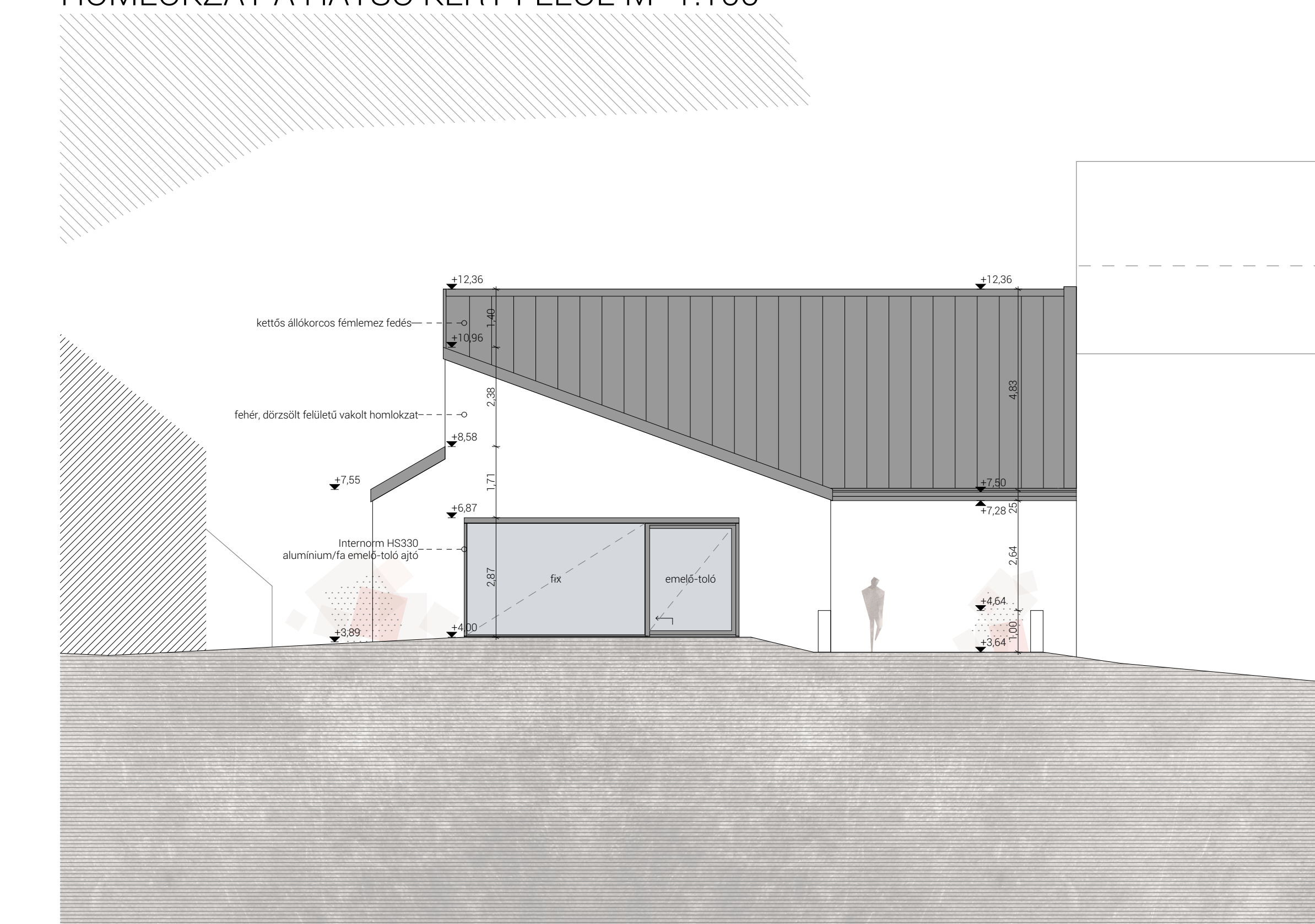
HOMLOKZAT A HÁTSÓ KERT FELŐL M=1:100
