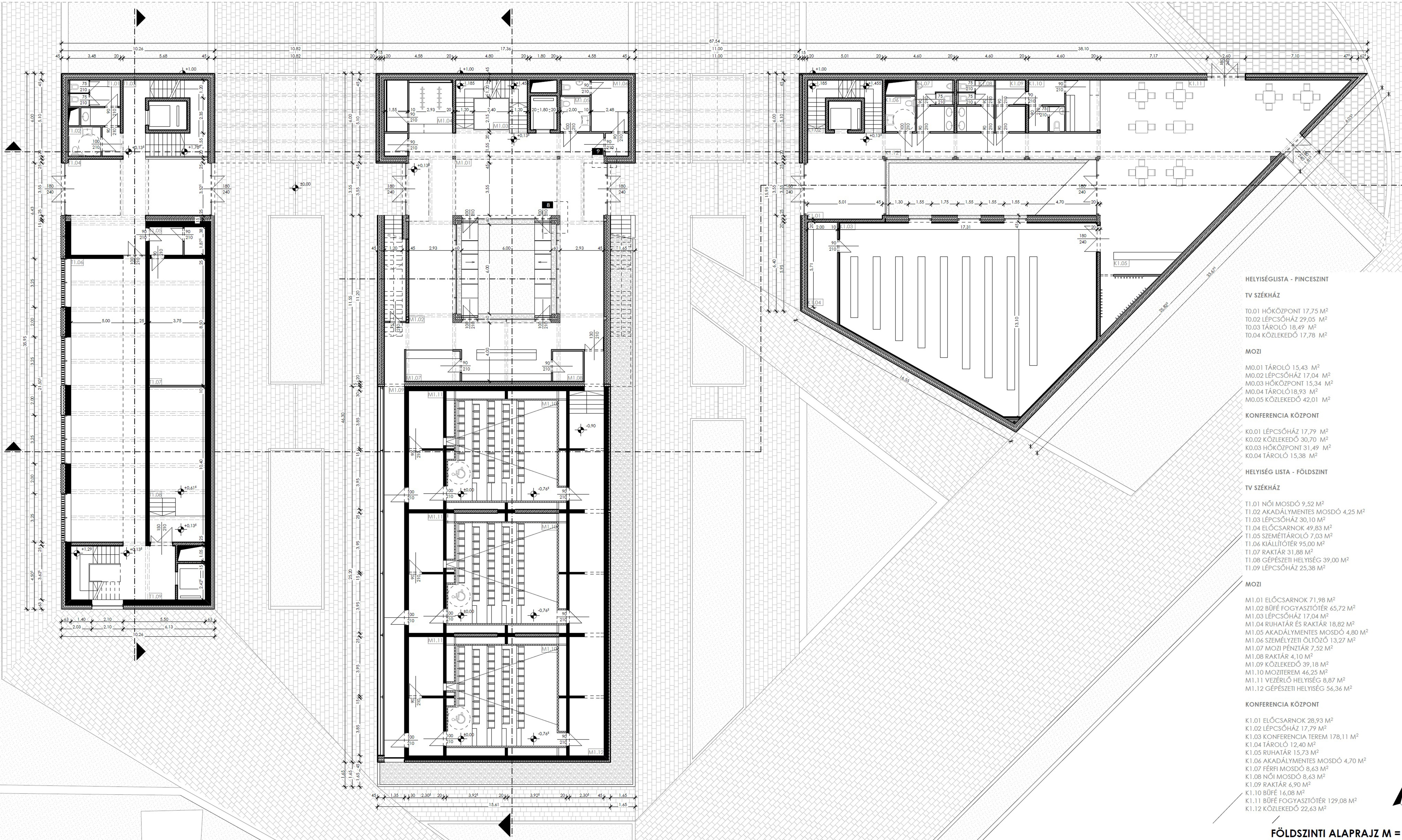
FÖLDSZINTI ALAPRAJZ M = 1:100
