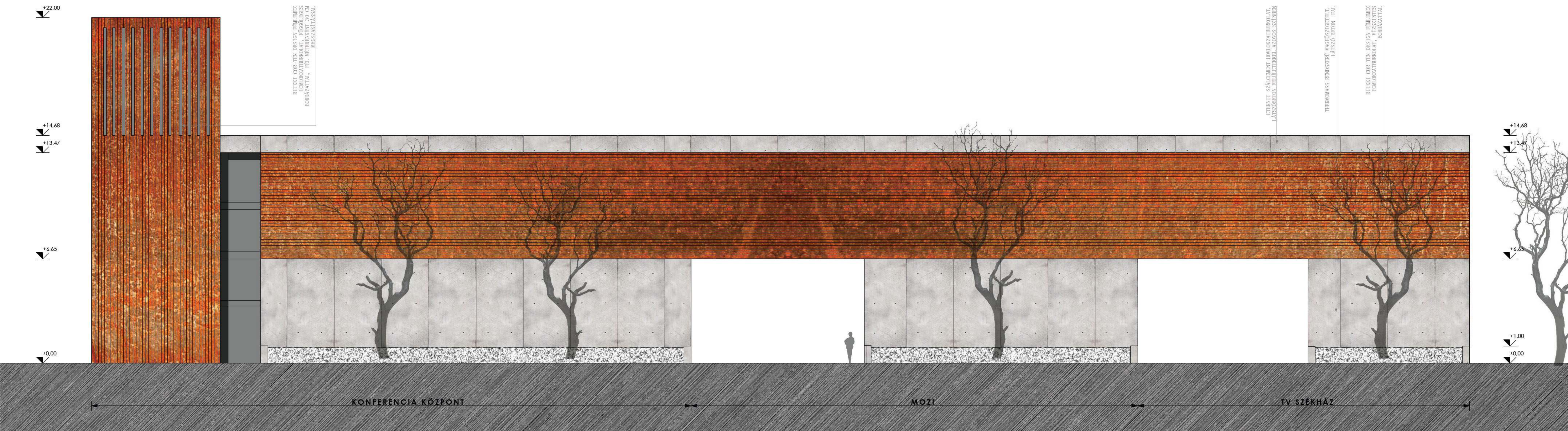
ÉSZAKI HOMLOKZAT M = 1:100
