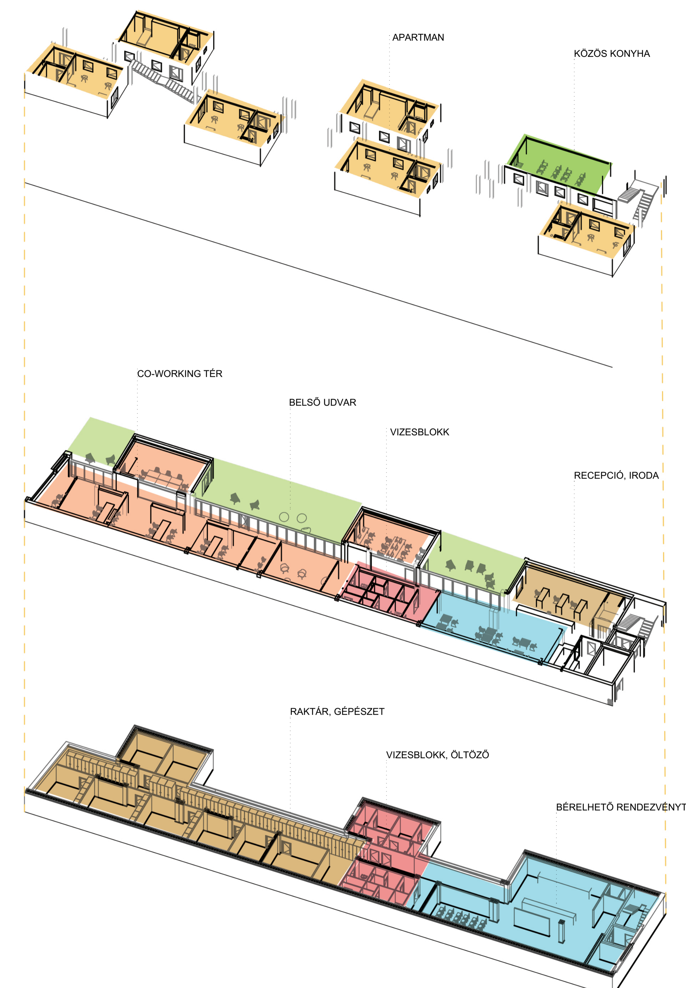
-1 szint alaprajz 1:100 DIÁKSZÁLLÓ SIMON ZSÓFIA JHZTAN LAKÓ // DIPLOMA 2020 JANUÁR 02
