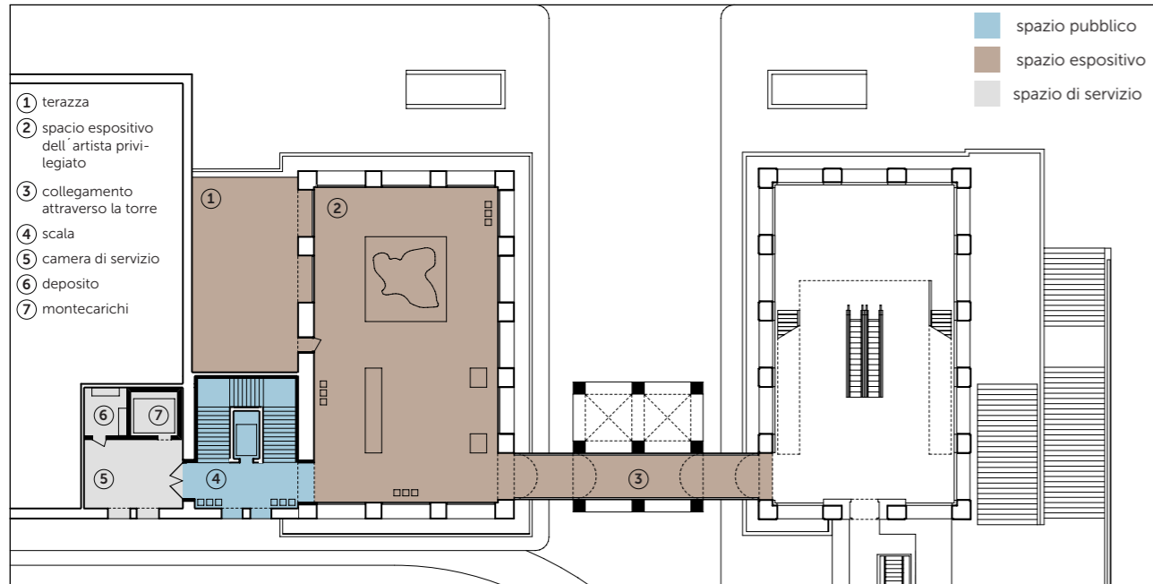
Pianta del 3° piano
