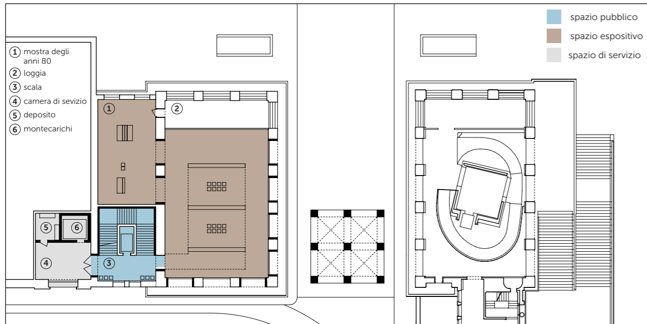
Pianta del 1° piano
