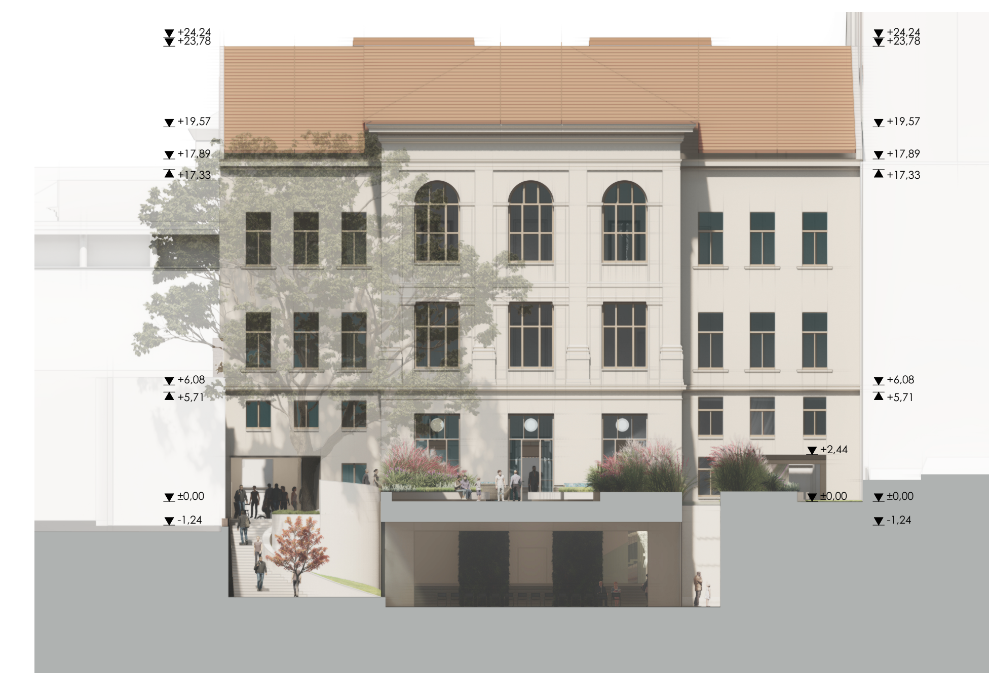
KELETI (UDVARI) HOMLOKZAT M1:200
