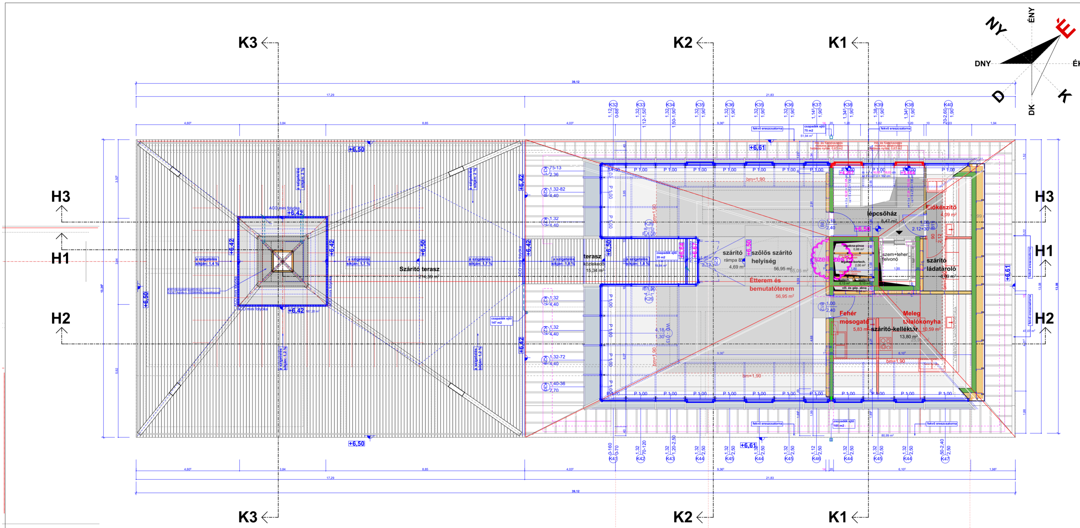
Tetőszinti alaprajz
