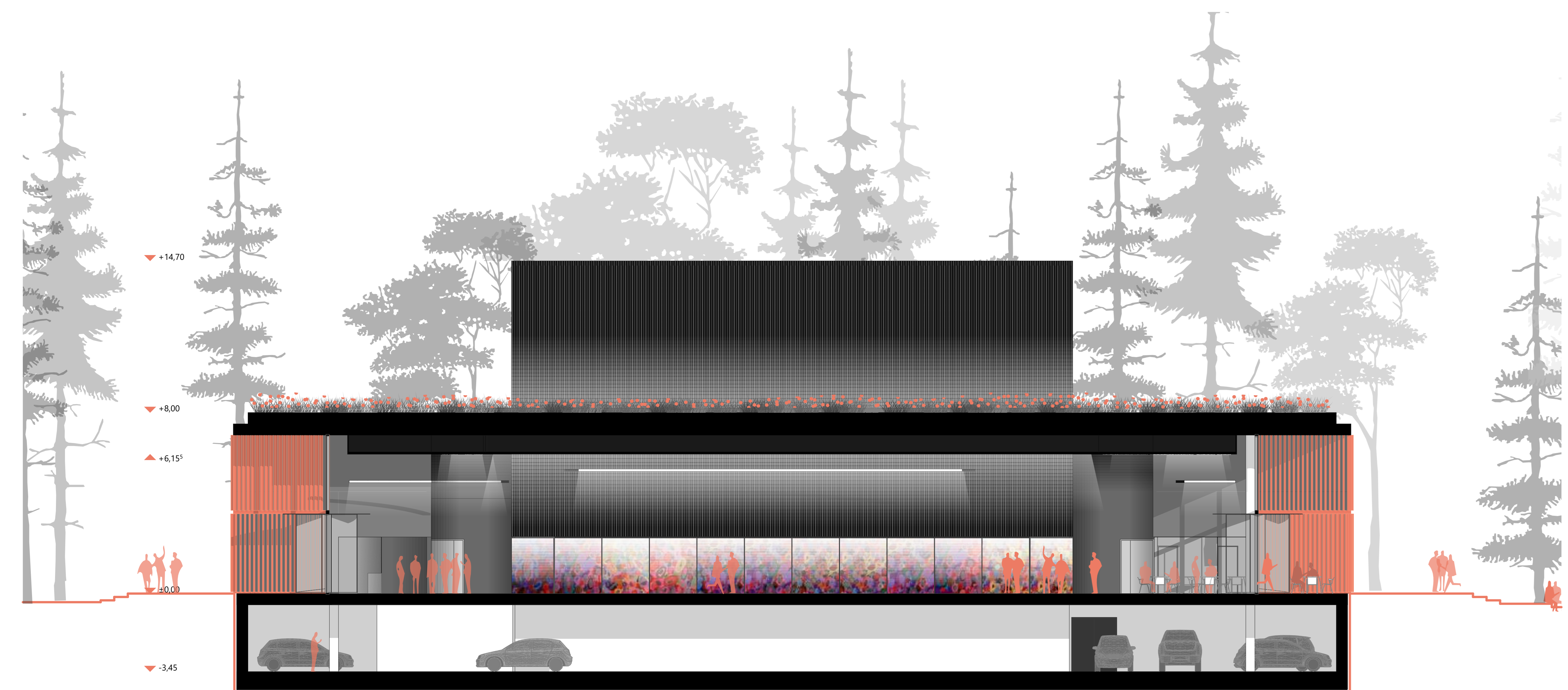
keresztmetszet _ előcsarnok
