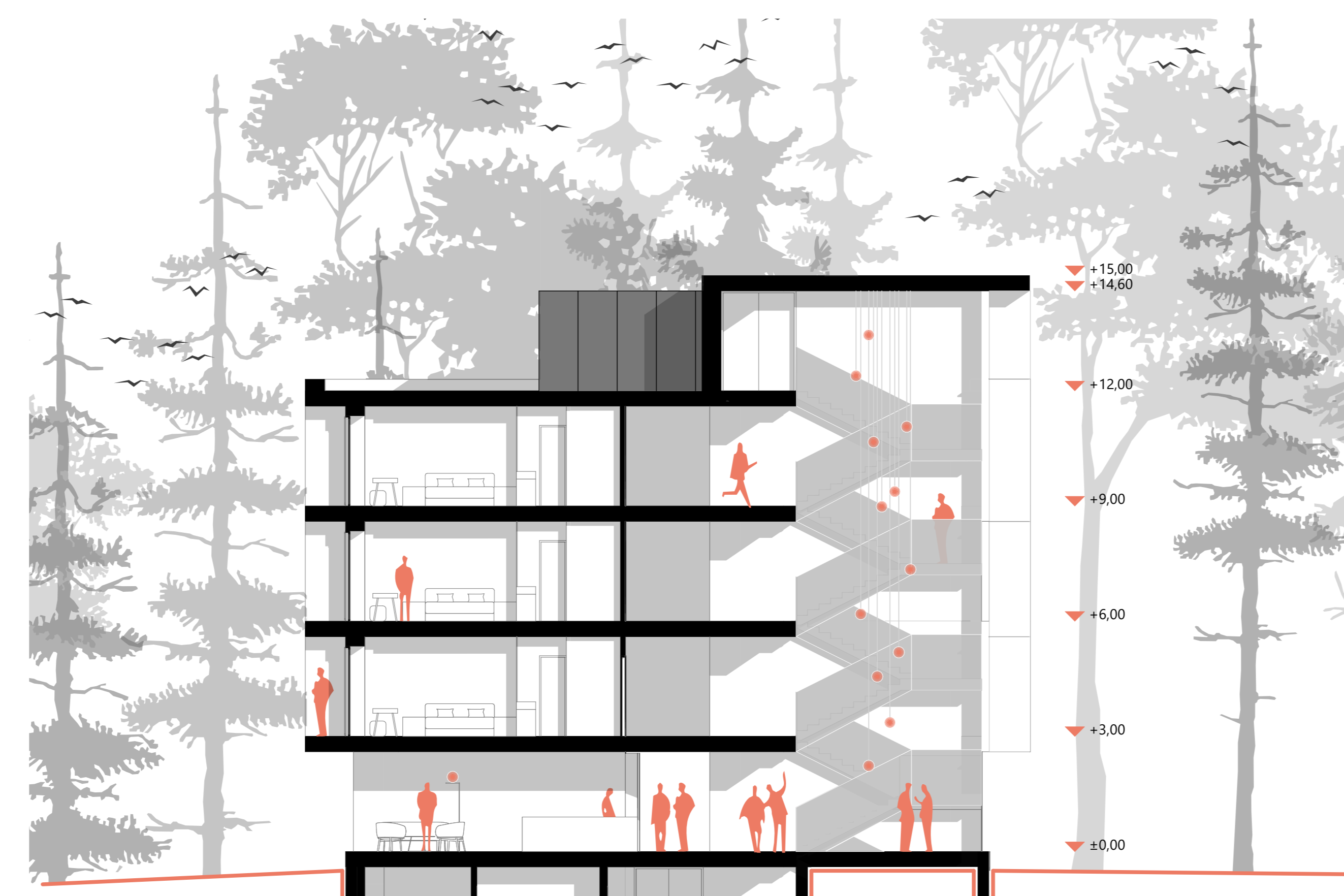
keresztmetszet
