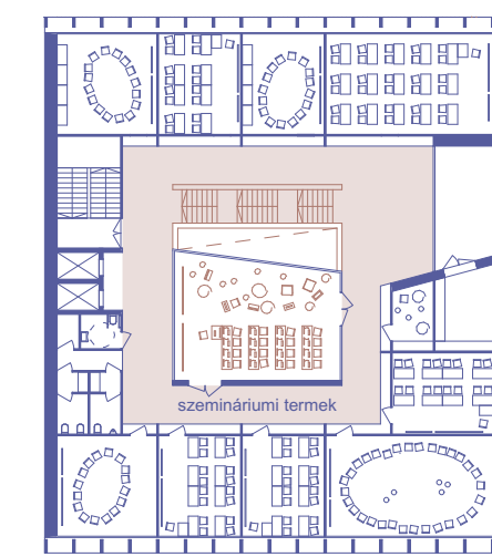
ÉSZAKI OKTATÁSI TORONY 2. emeleti alaprajz 1:500
