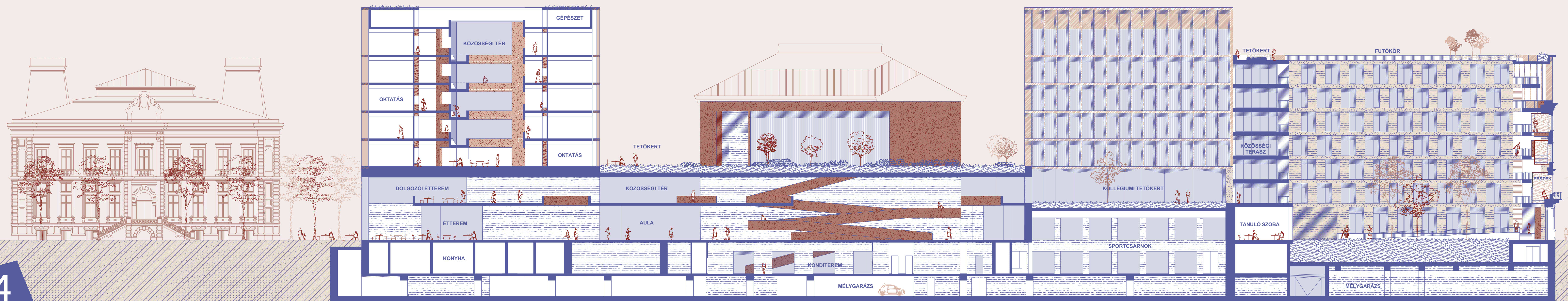
*A* HOSSZMETSZET a tanulási tájon és a kollégiumon keresztül 1:250
