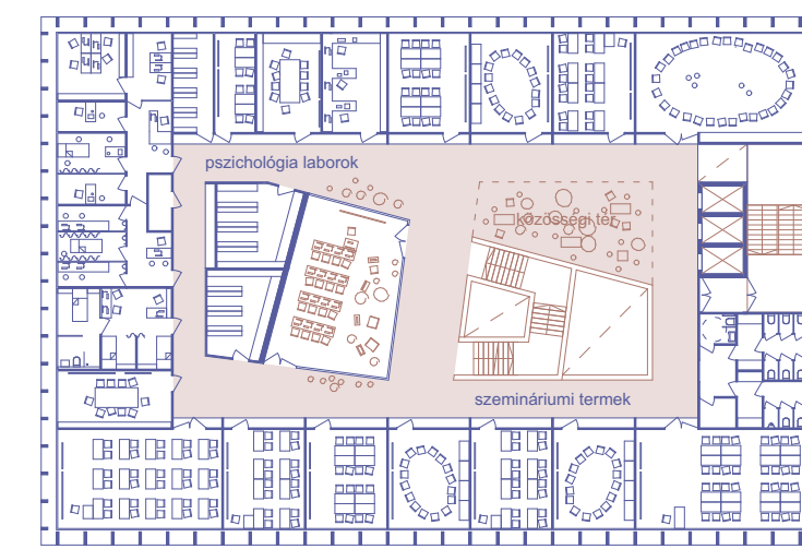
KELETI OKTATÁSI TORONY 4. emeleti alaprajz 1:500
