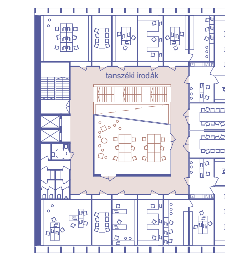
ÉSZAKI OKTATÁSI TORONY 5. emeleti alaprajz 1:500
