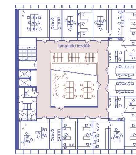
ÉSZAKI OKTATÁSI TORONY 3. emeleti alaprajz 1:500
