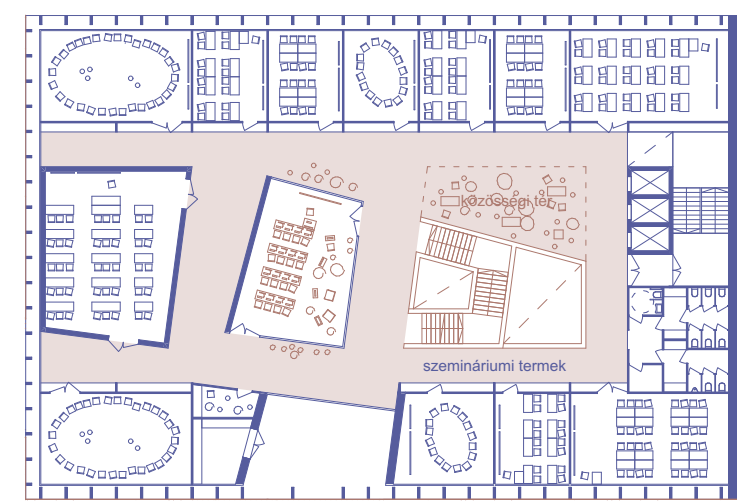
KELETI OKTATÁSI TORONY 2. emeleti alaprajz 1:500
