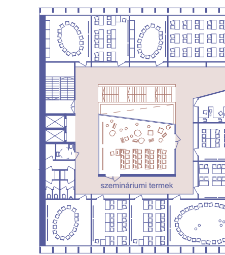
ÉSZAKI OKTATÁSI TORONY 6. emeleti alaprajz 1:500
