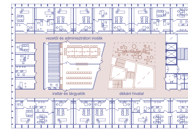
KELETI OKTATÁSI TORONY 5. emeleti alaprajz 1:500
