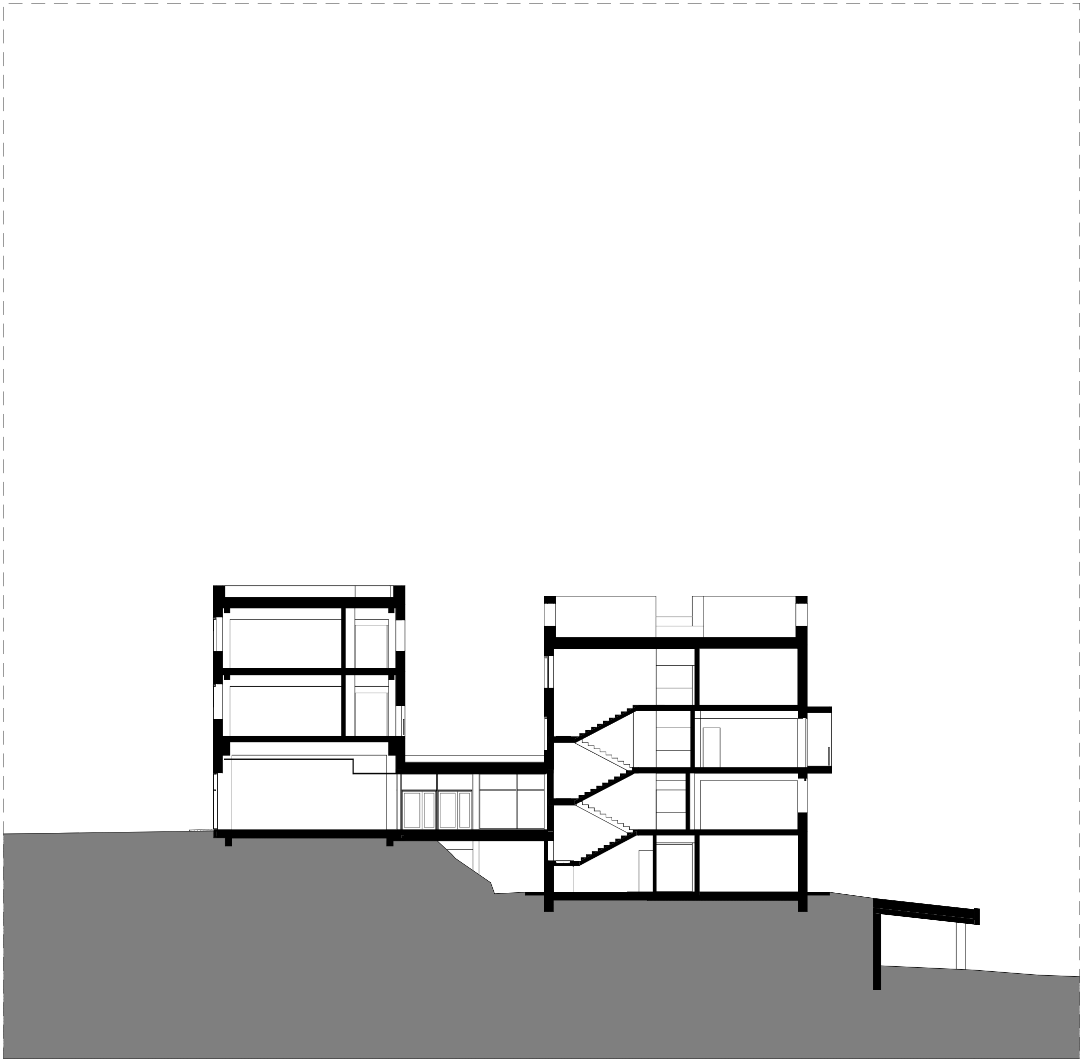
A-A METSZET
