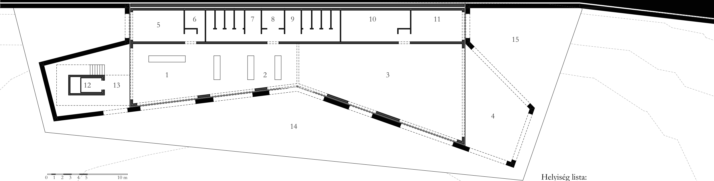
Udvarszinti alaprajz 1:200
