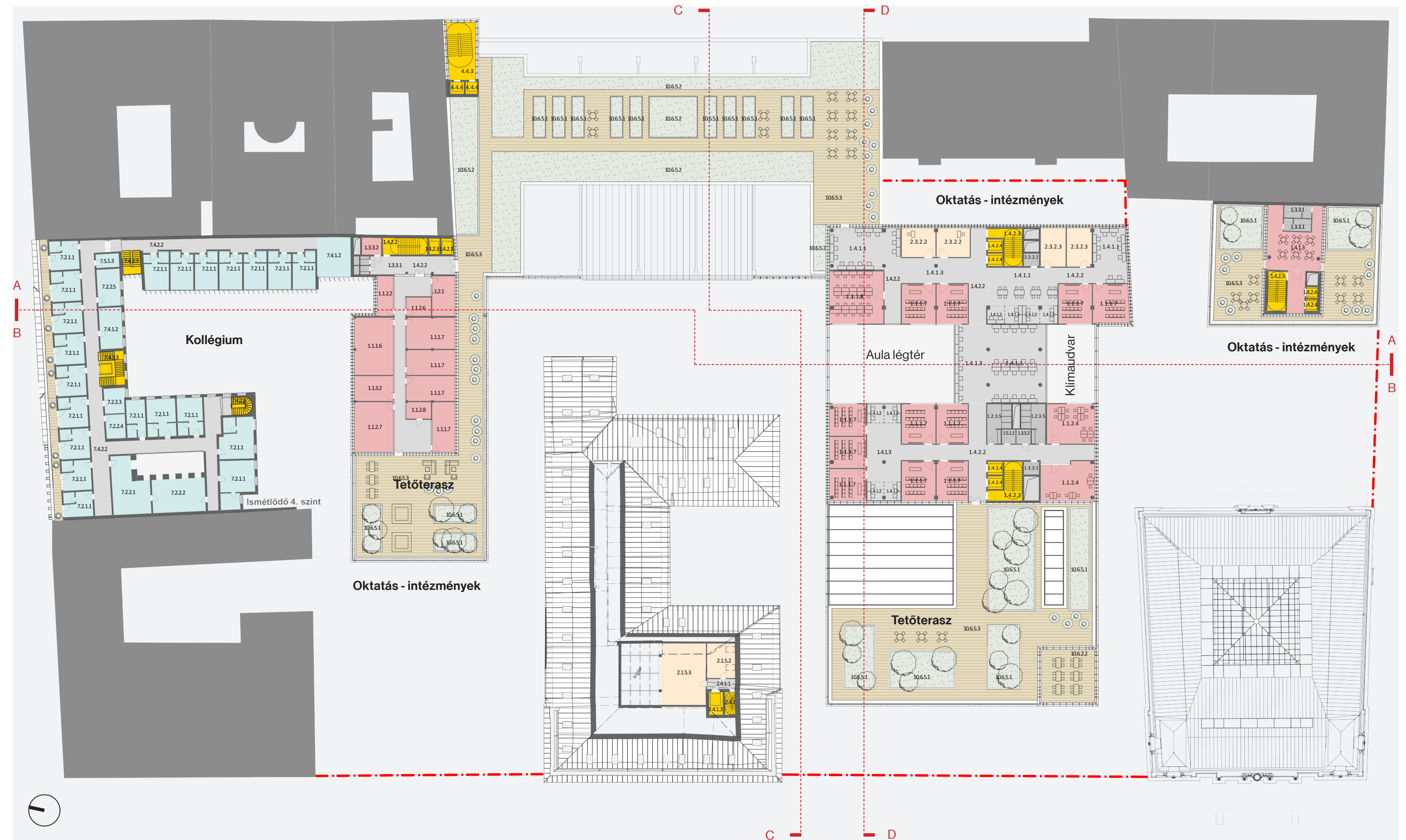
HATODIK EMELETI ALAPRAJZ · 1:500
