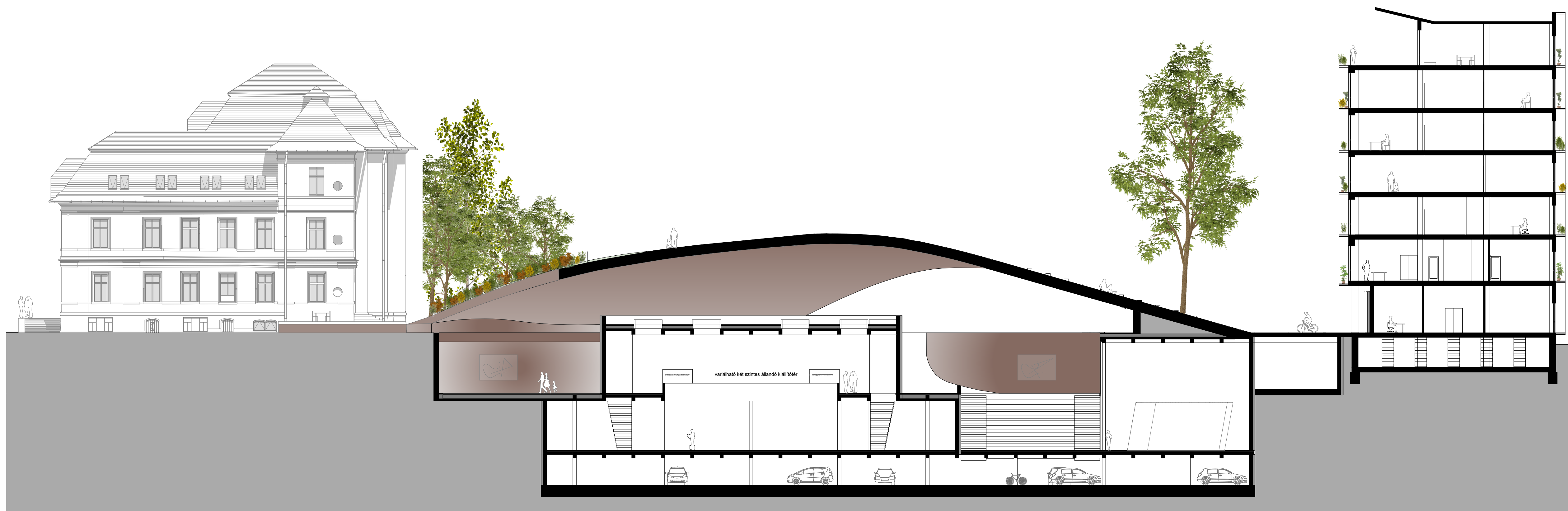
B-B METSZET M=1:200
