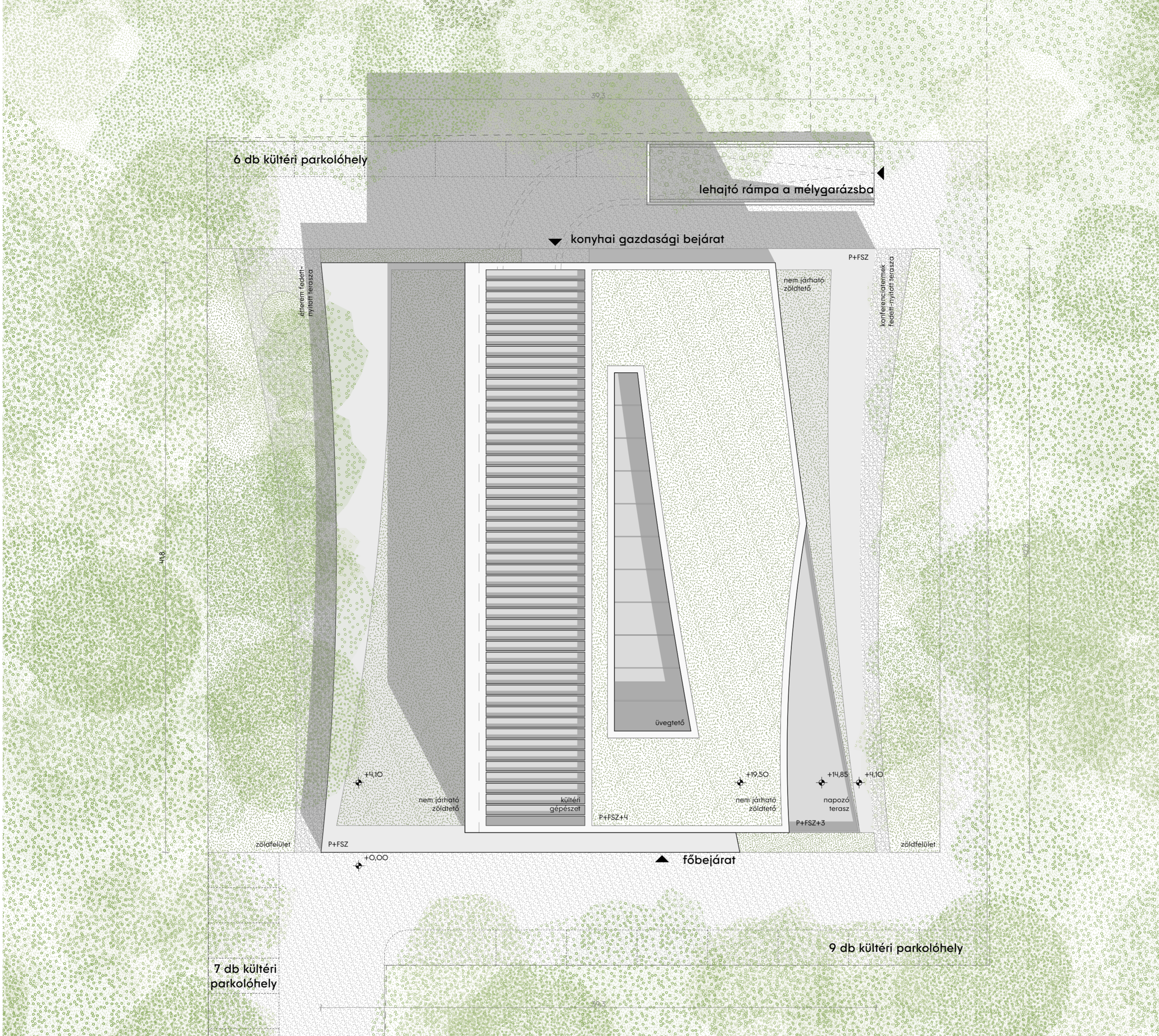
1 tetőfelülnézet - m 1:200
