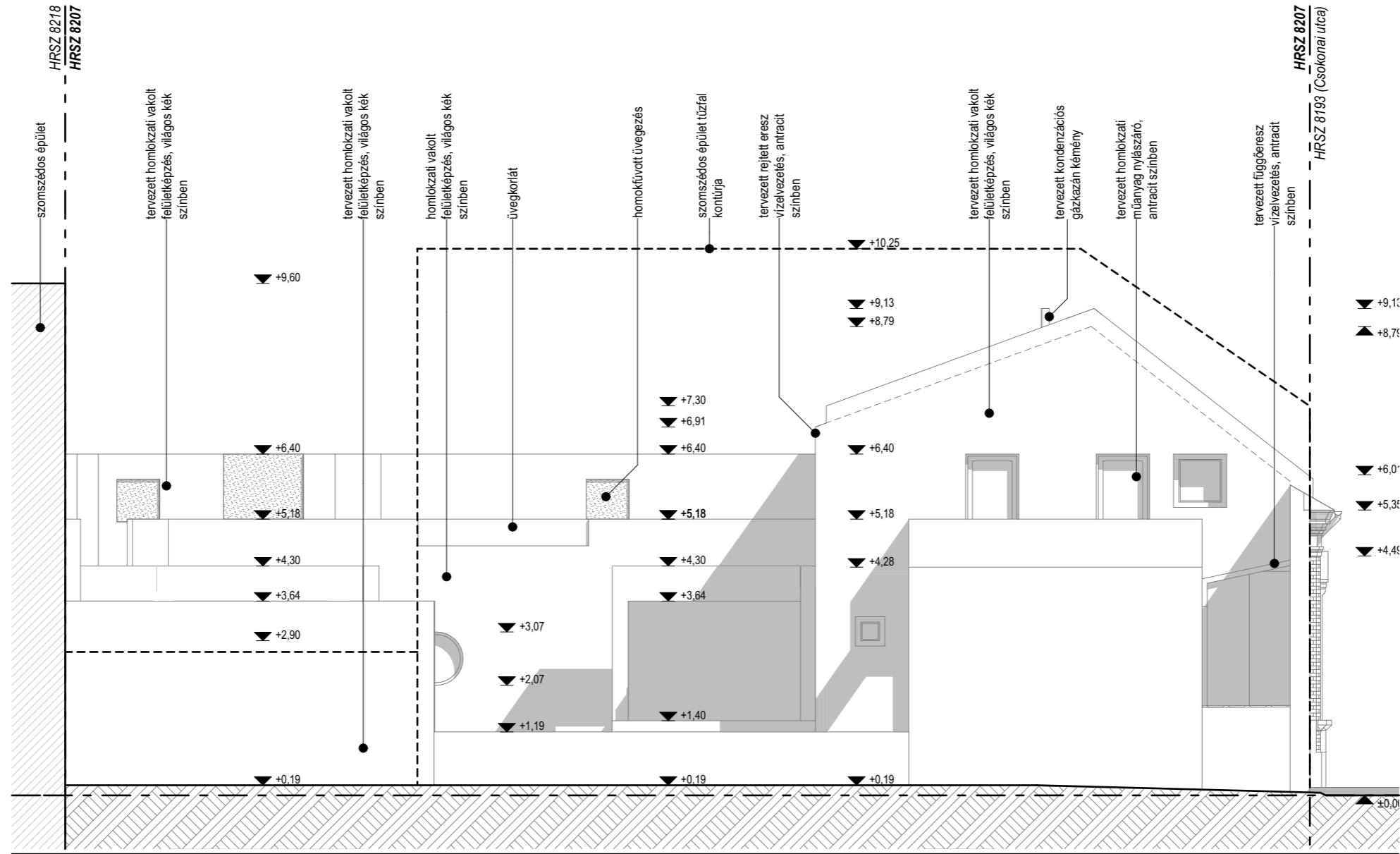
4. Homlokzat M=1:100
