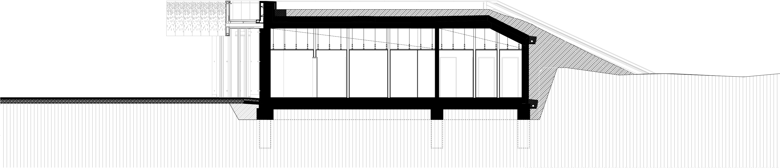
B-B METSZET
