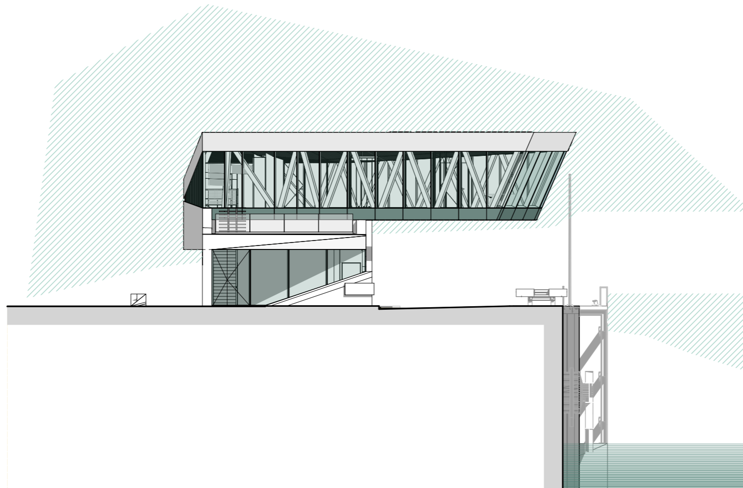
0 1 5 KELETI HOMLOKZAT
