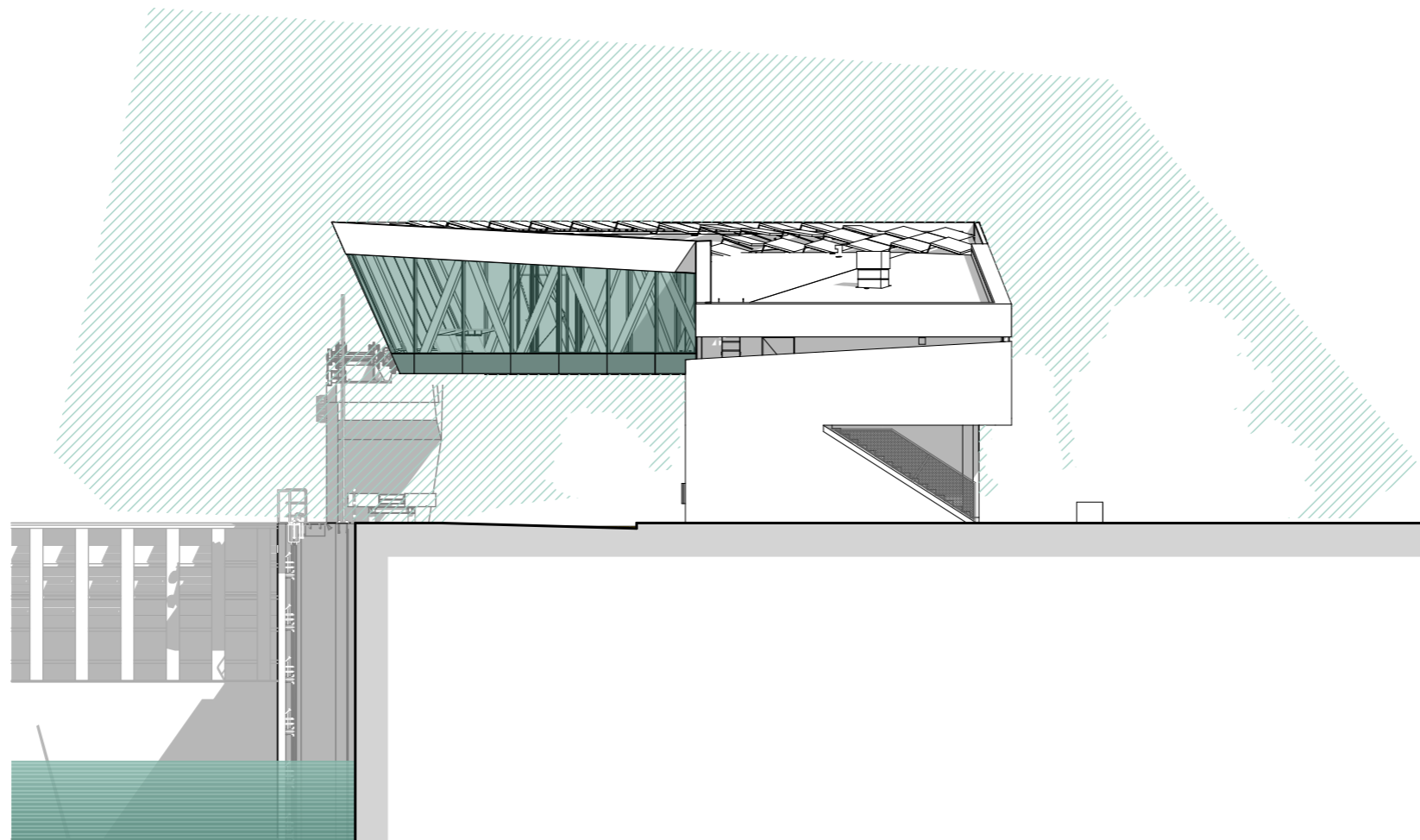
0 1 5 NYUGATI HOMLOKZAT
