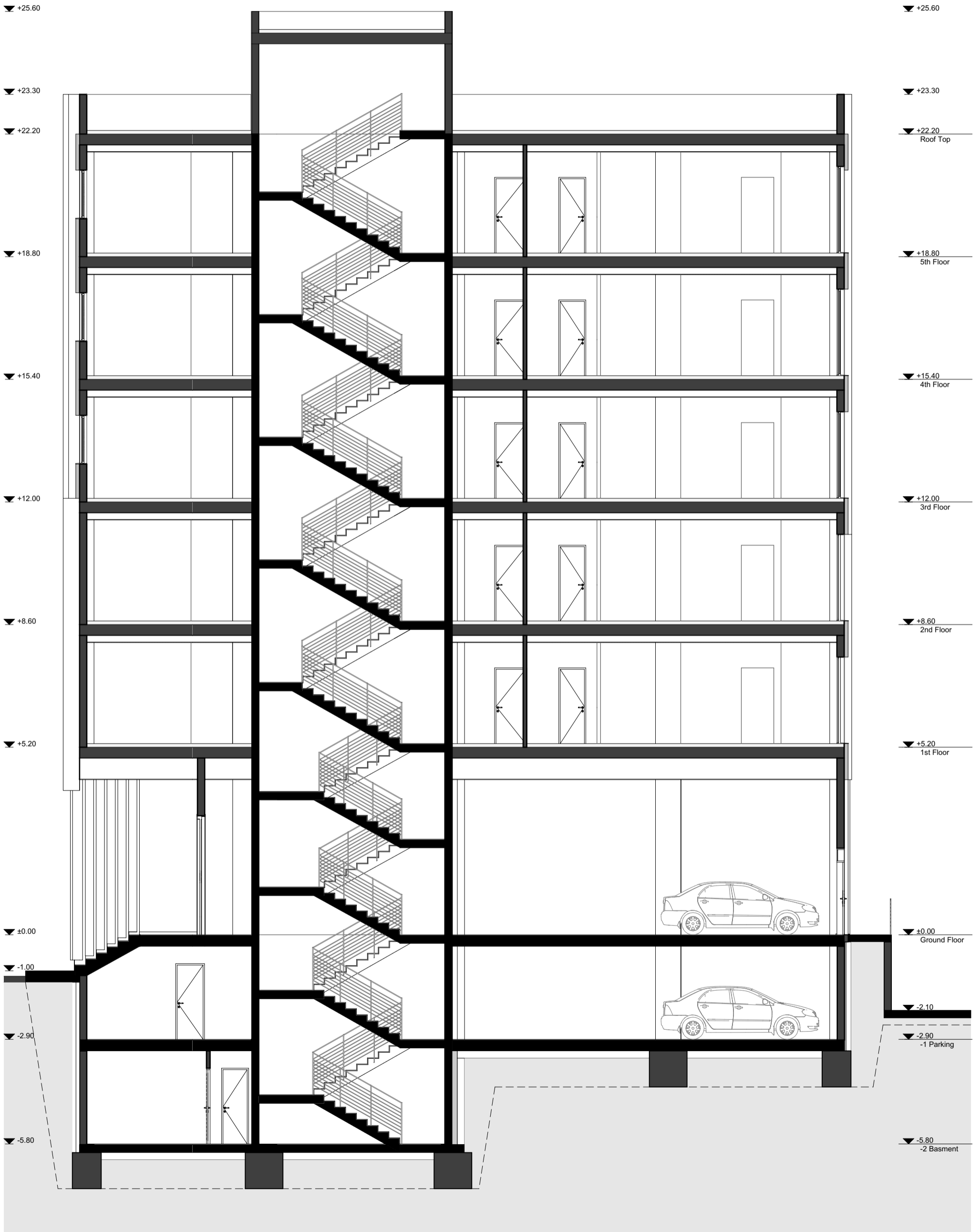
Section A-A
