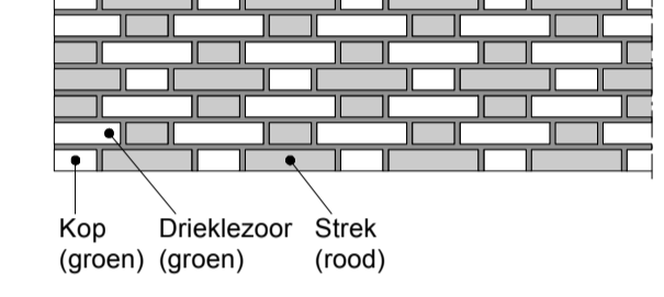
Metselwerk patroon B - Fragment schaal 1:20
