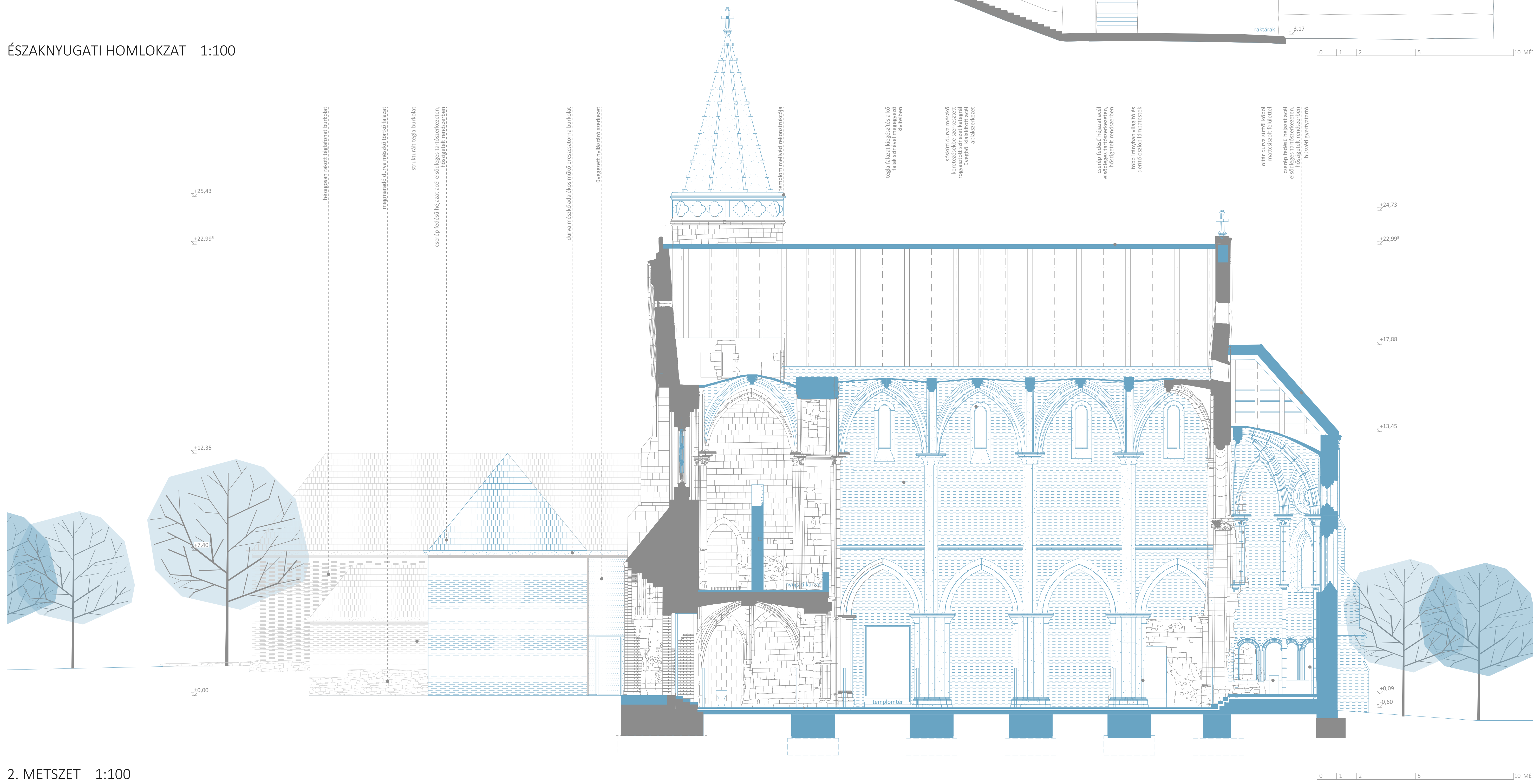
2. METSZET 1:100
