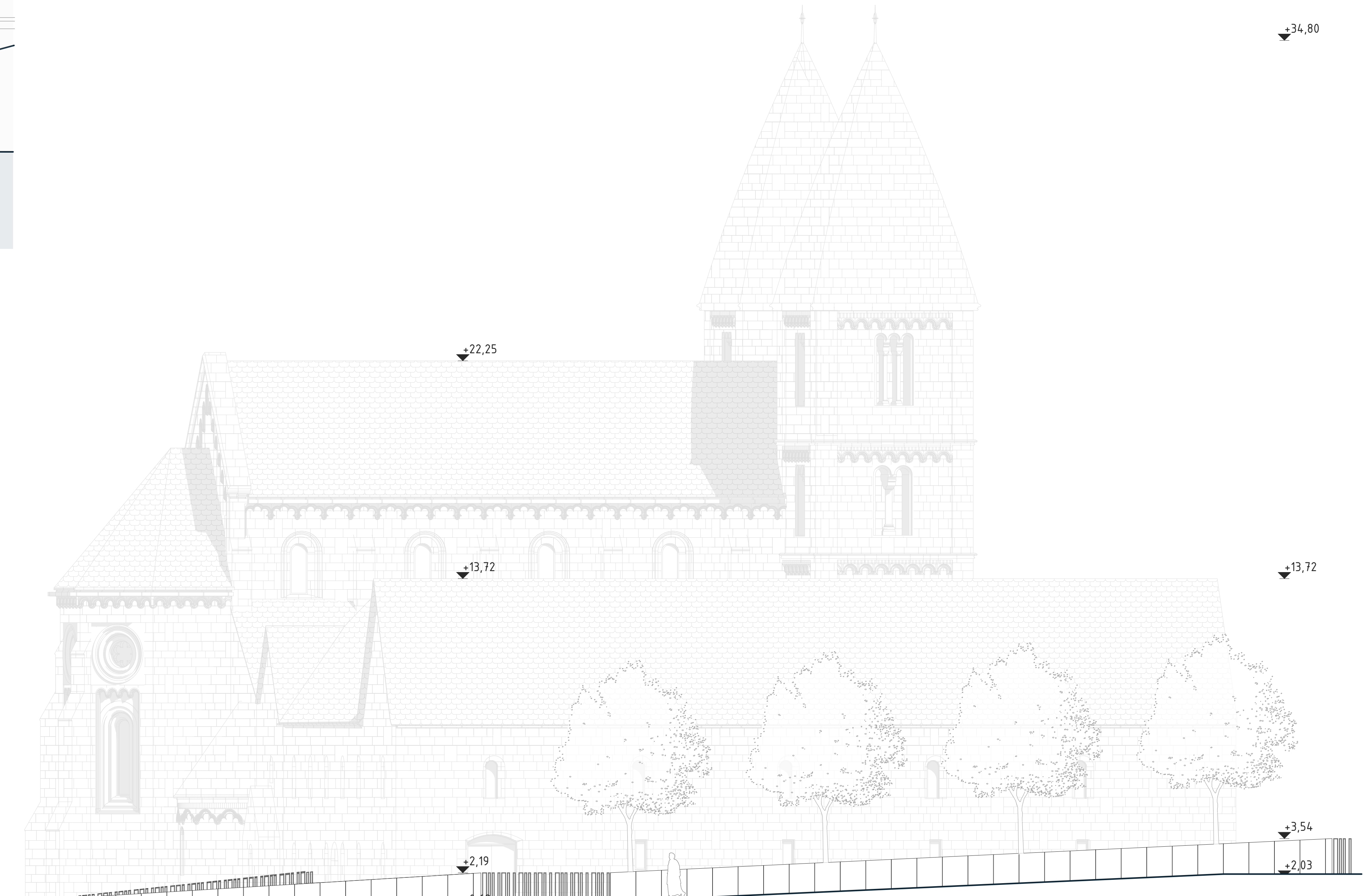
ÉSZAKI HOMLOKZAT M=1:100
