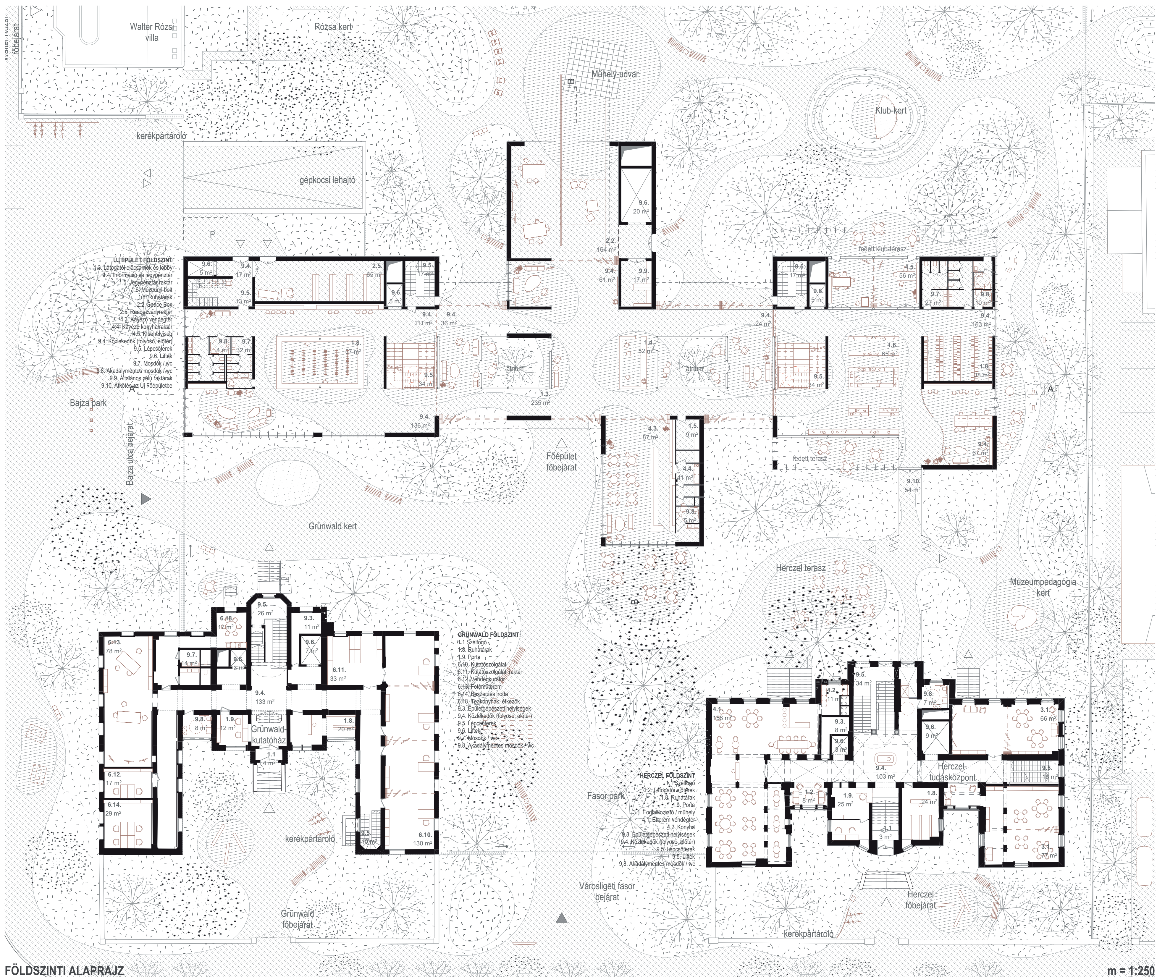
FÖLDSZINTI ALAPRAJZ
