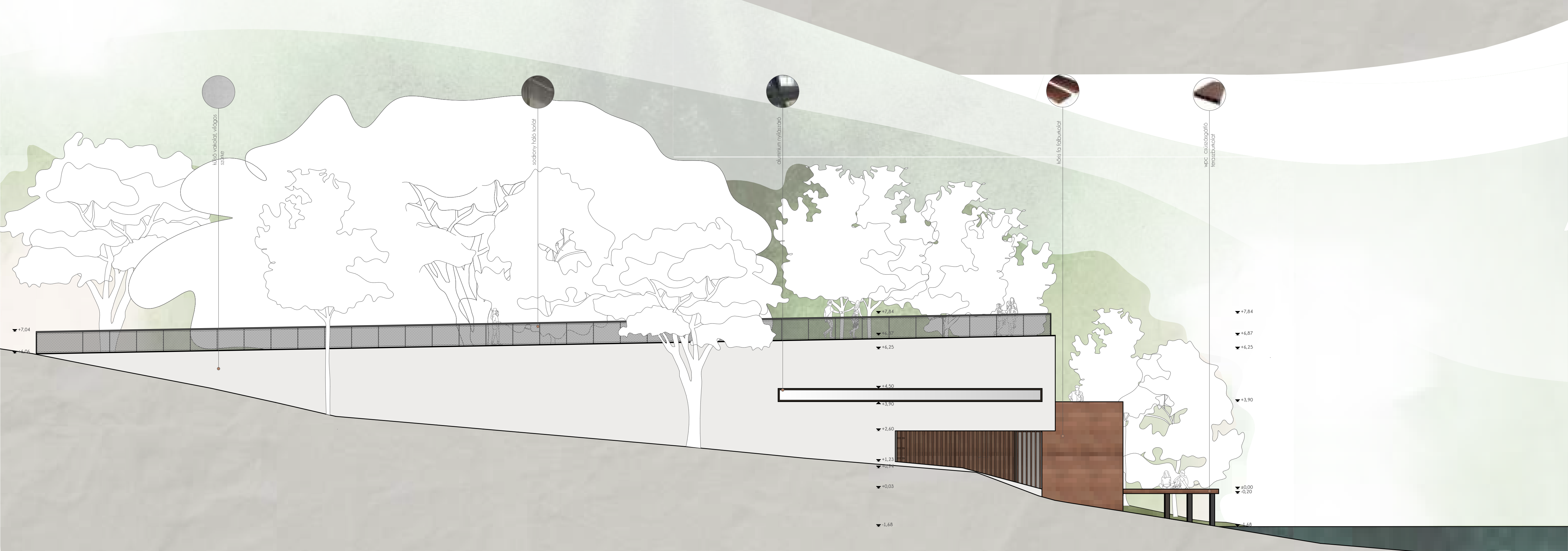
Déli Homlokzat M1:100
