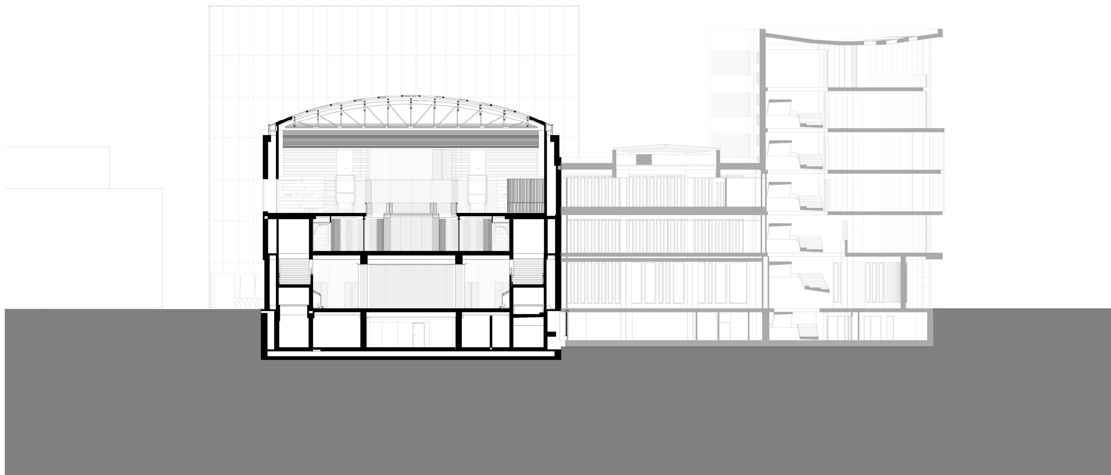
A-A metszet
