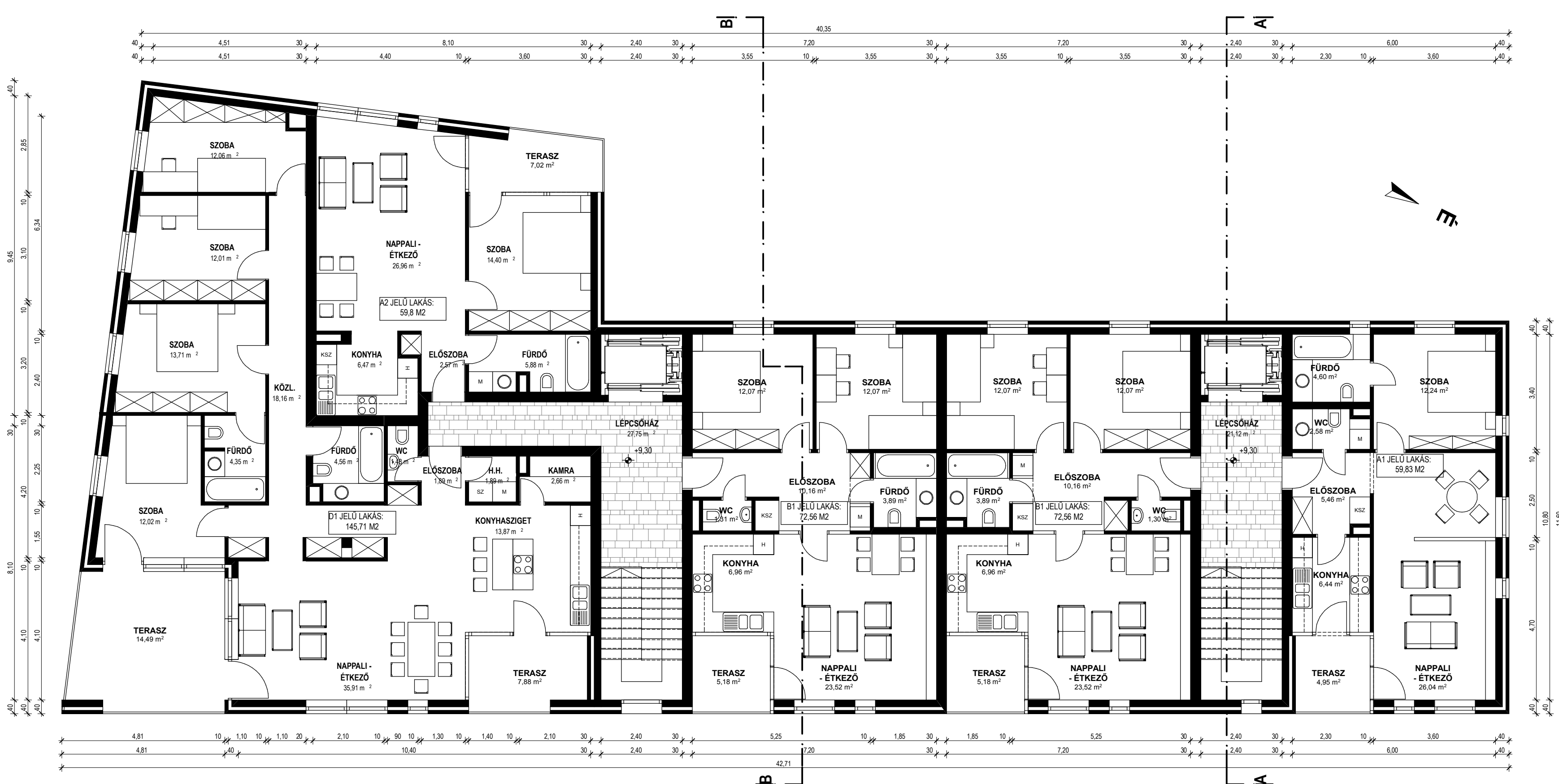
III-IV. EMELETI ALAPRAJZ M 1:100
