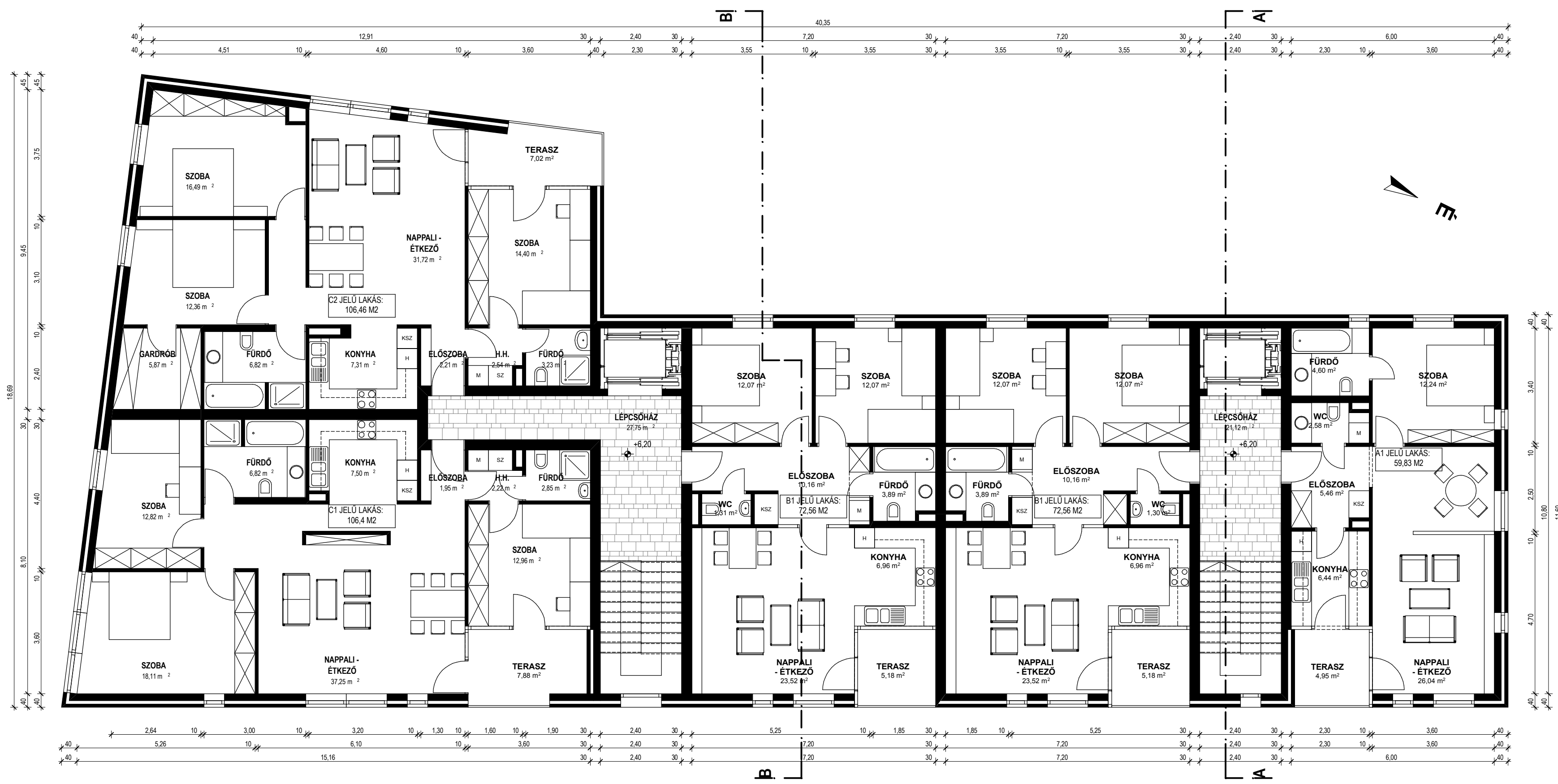
II. EMELETI ALAPRAJZ M 1:100
