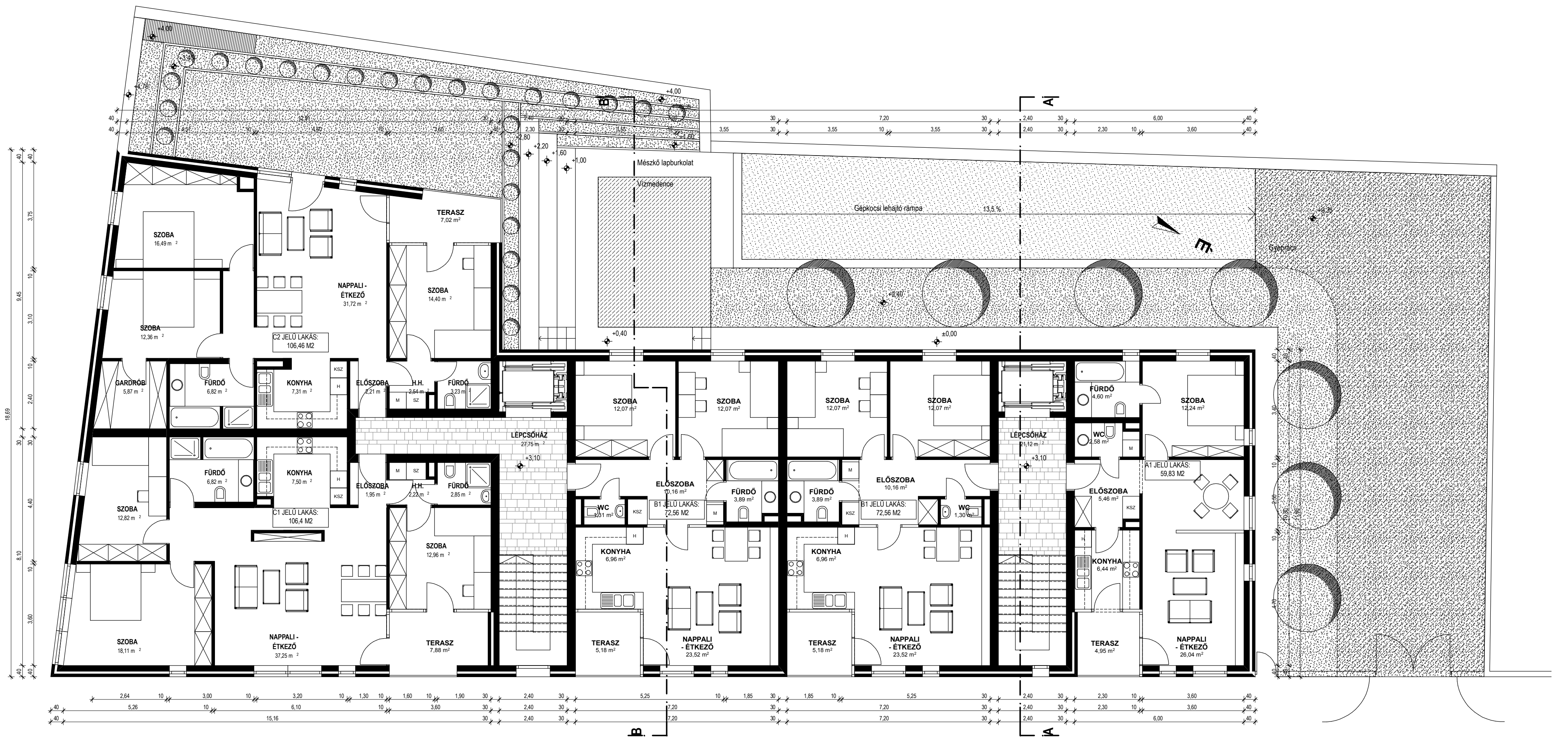
I. EMELETI ALAPRAJZ M 1:100
