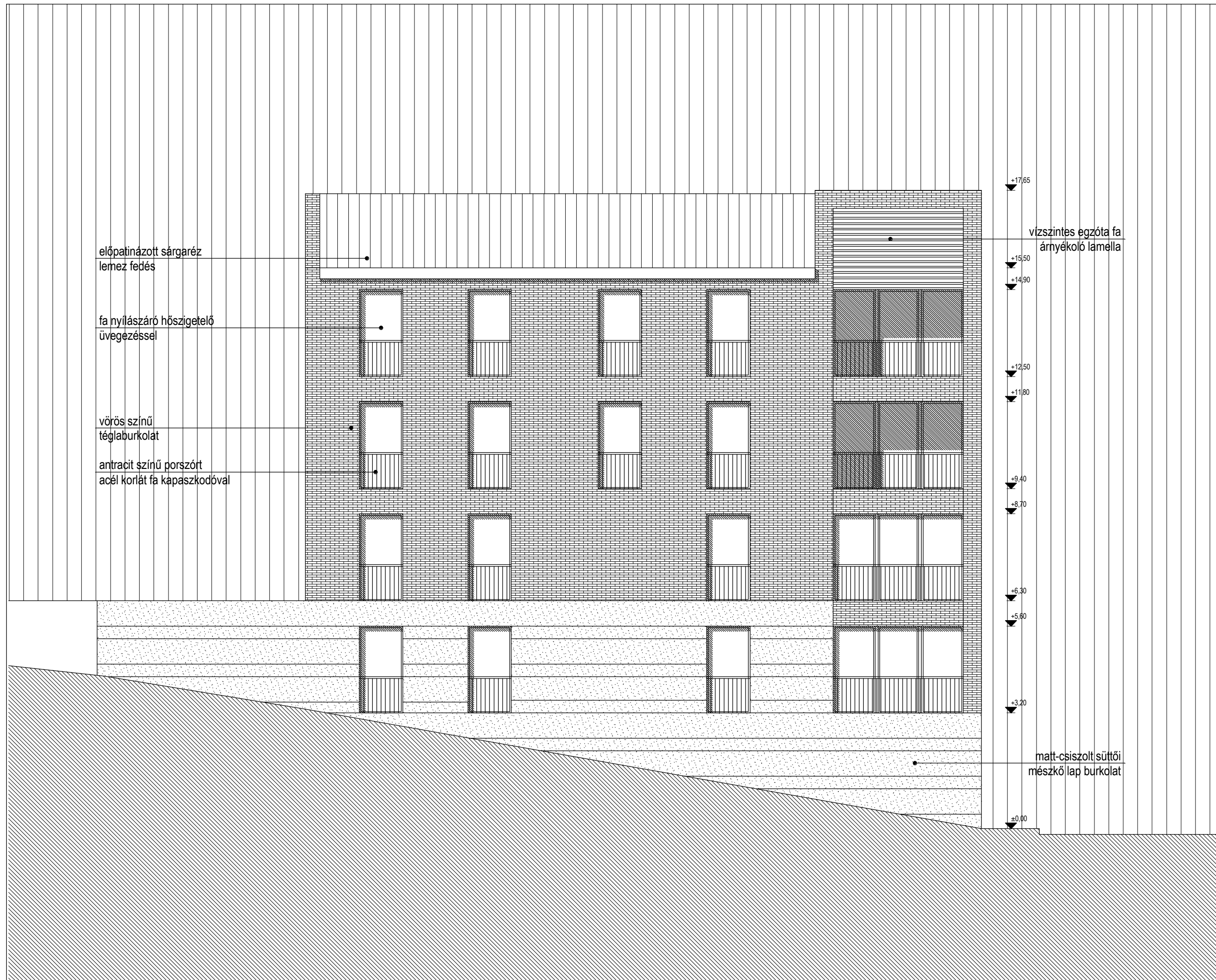
DÉLI HOMLOKZAT M 1:100
