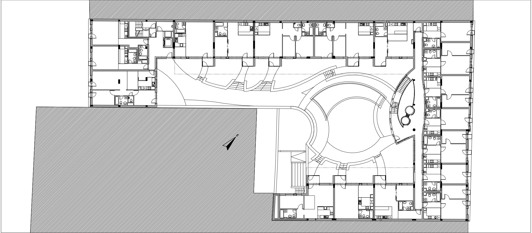
AKÁCFA UTCA 12-14. - 1. EMELETI ALAPRAJZ
