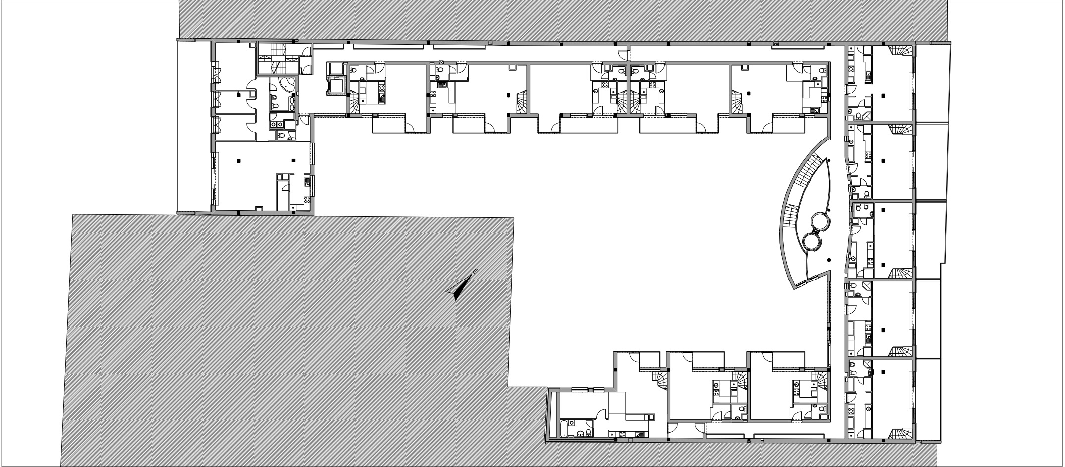
AKÁCSFA UTCA 12-14. - TETŐTÉRI ALAPRAJZ
