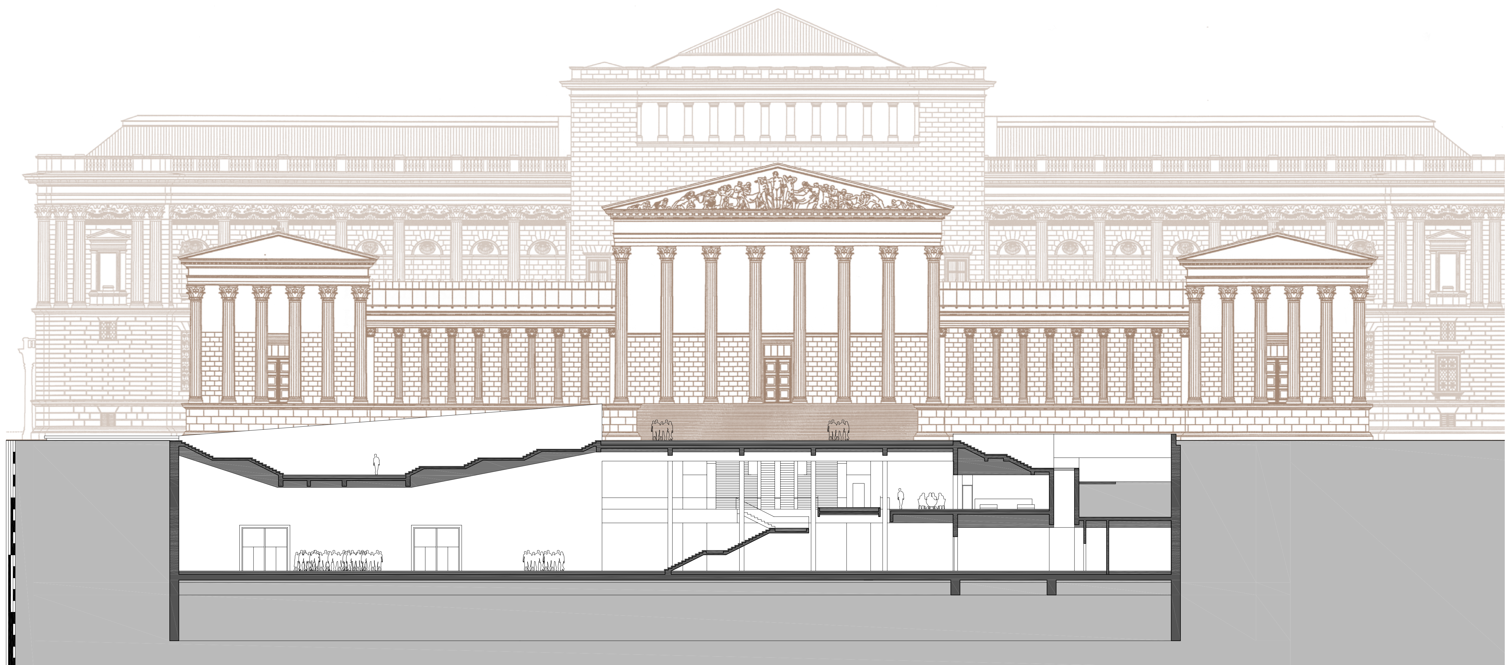
metszet az előcsarnokon keresztül
