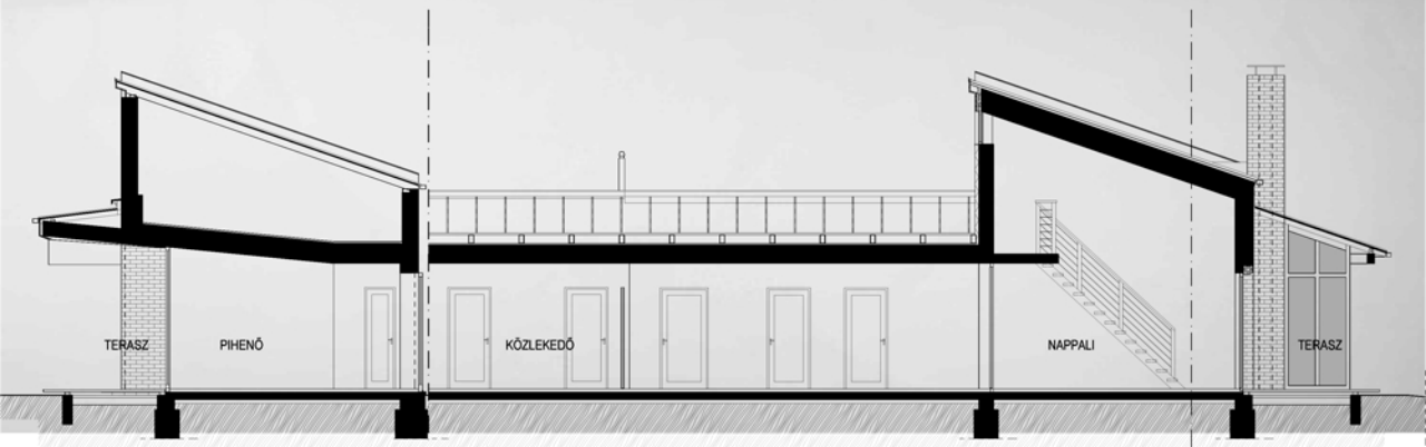
A - A METSZET M 1:100
