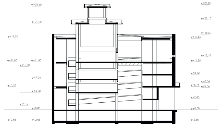
B-B metszet
