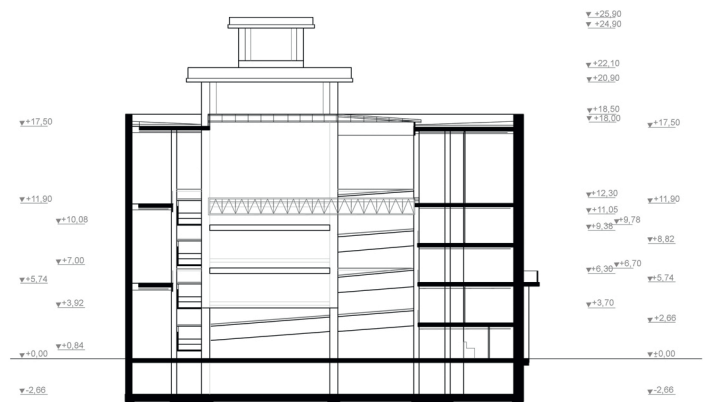
D-D metszet
