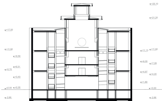
A-A metszet
