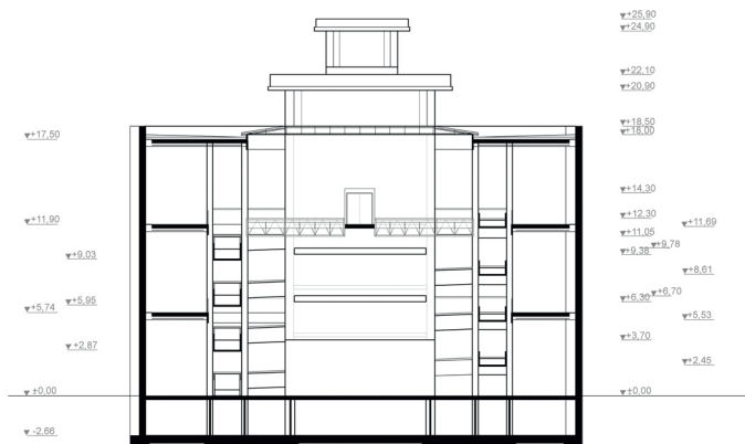
C-C metszet
