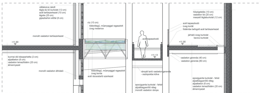
A-A metszet M 1:50
