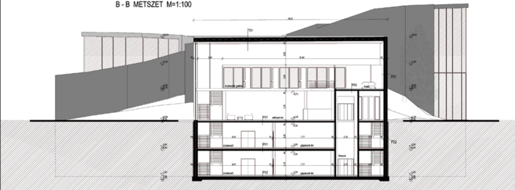
B - B METSZET M=1:100
