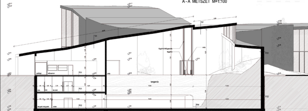
A - A METSZET M=1:100
