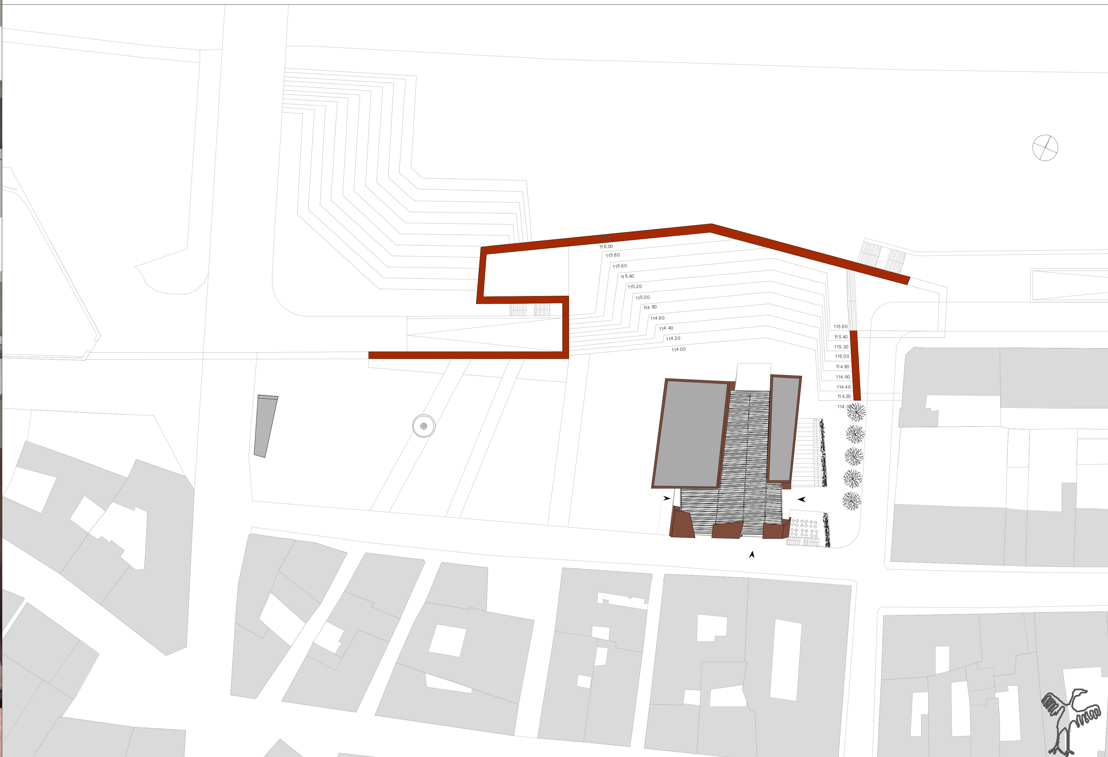
A DUNAKAPU TÉR DÉLI TÉRFALA A TÉRÜJ ÉPÜLETÉVEL M 1: 500
