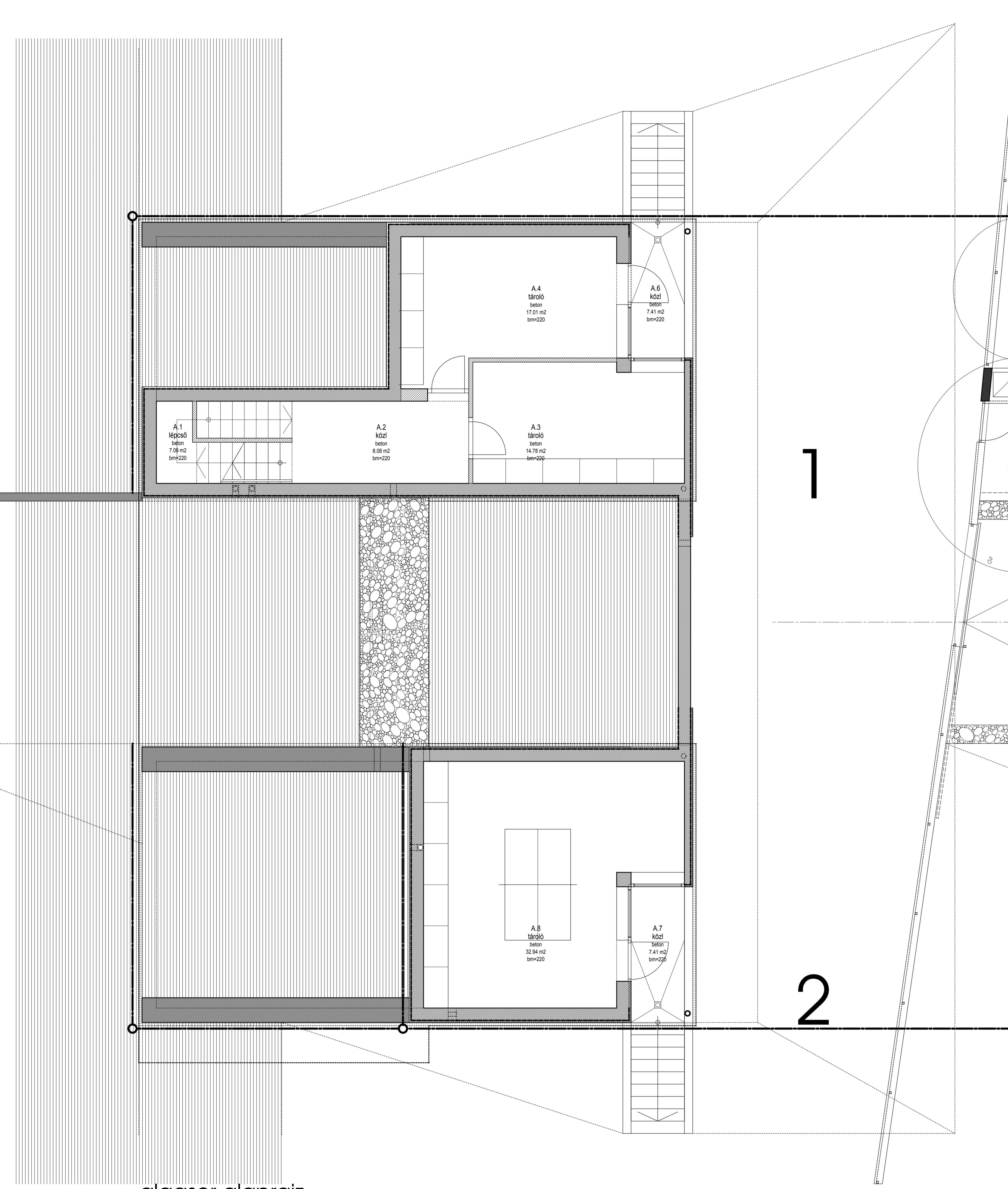
alagsor alaprajz
