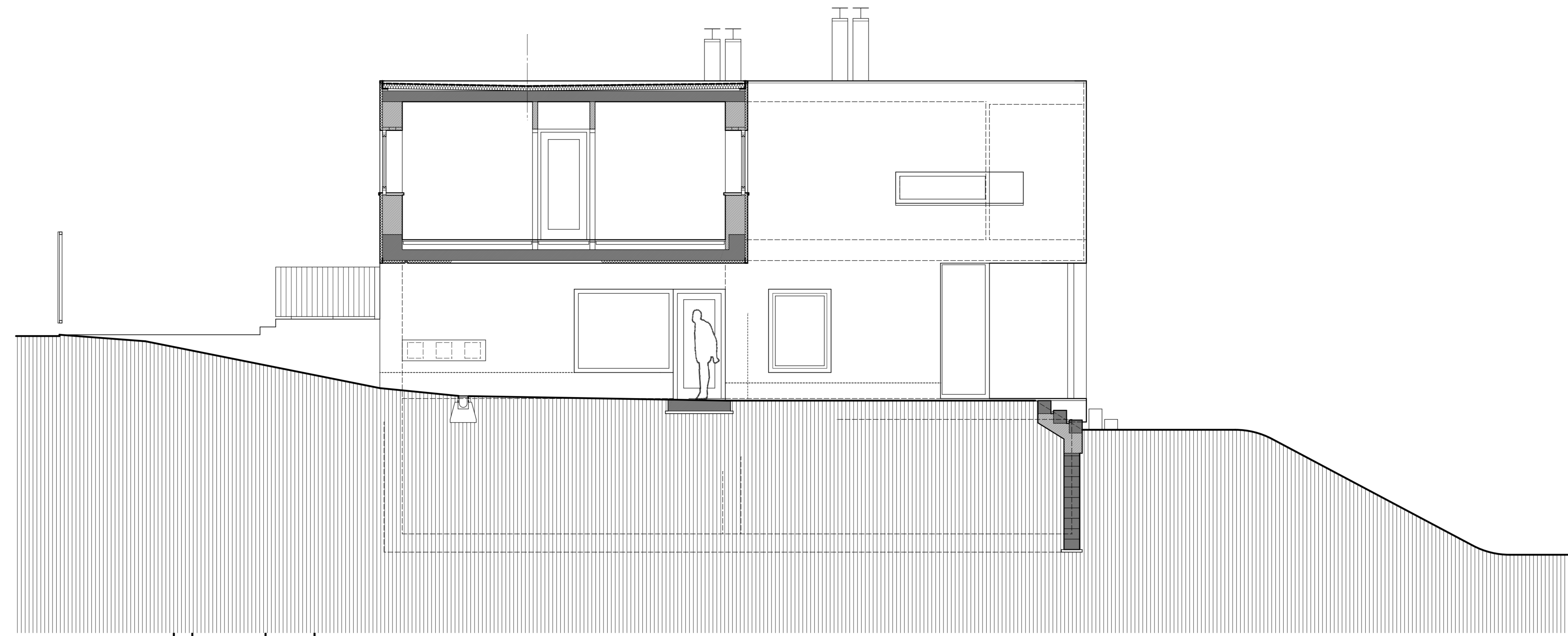
bb metszet
