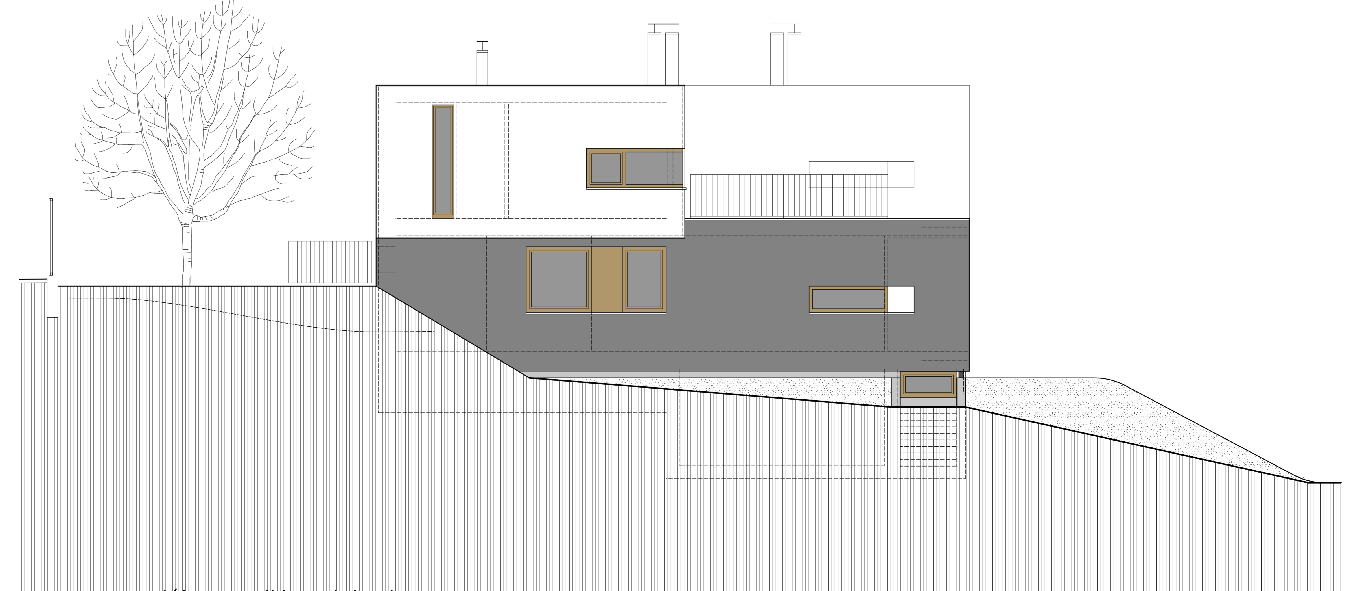
dél-nyugati homlokzat
