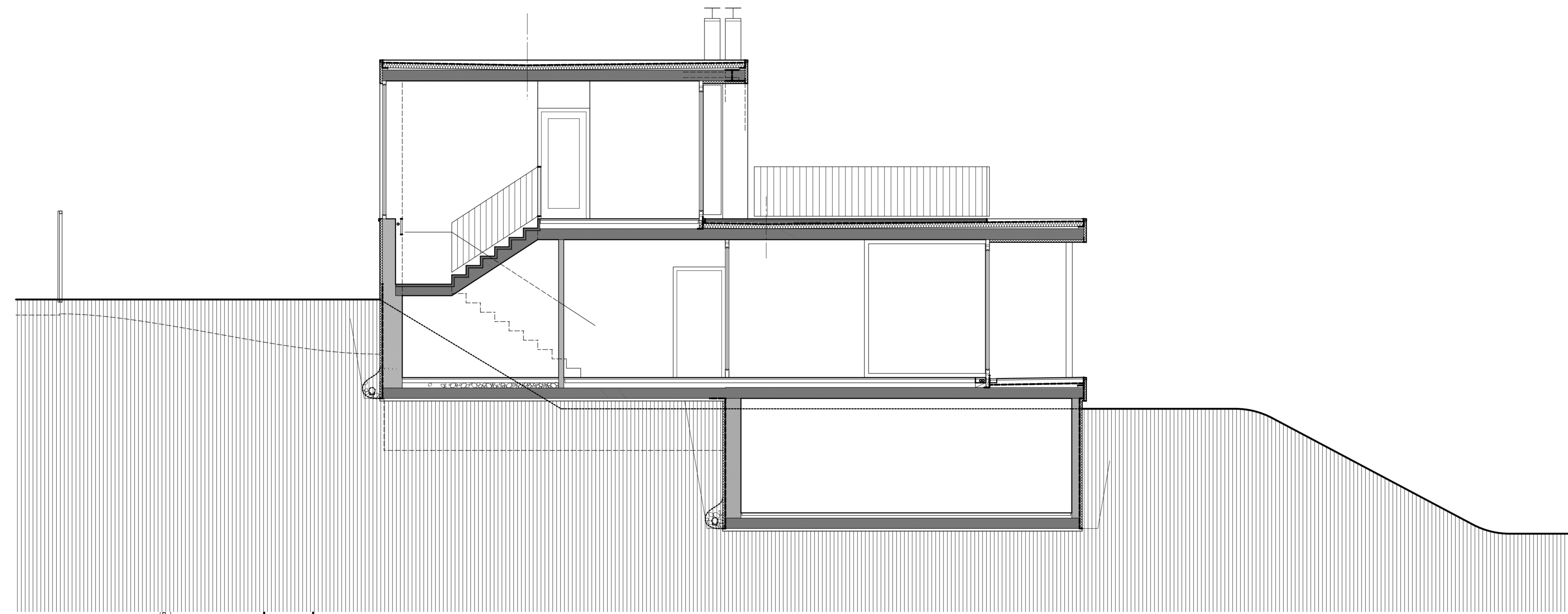
cc metszet
