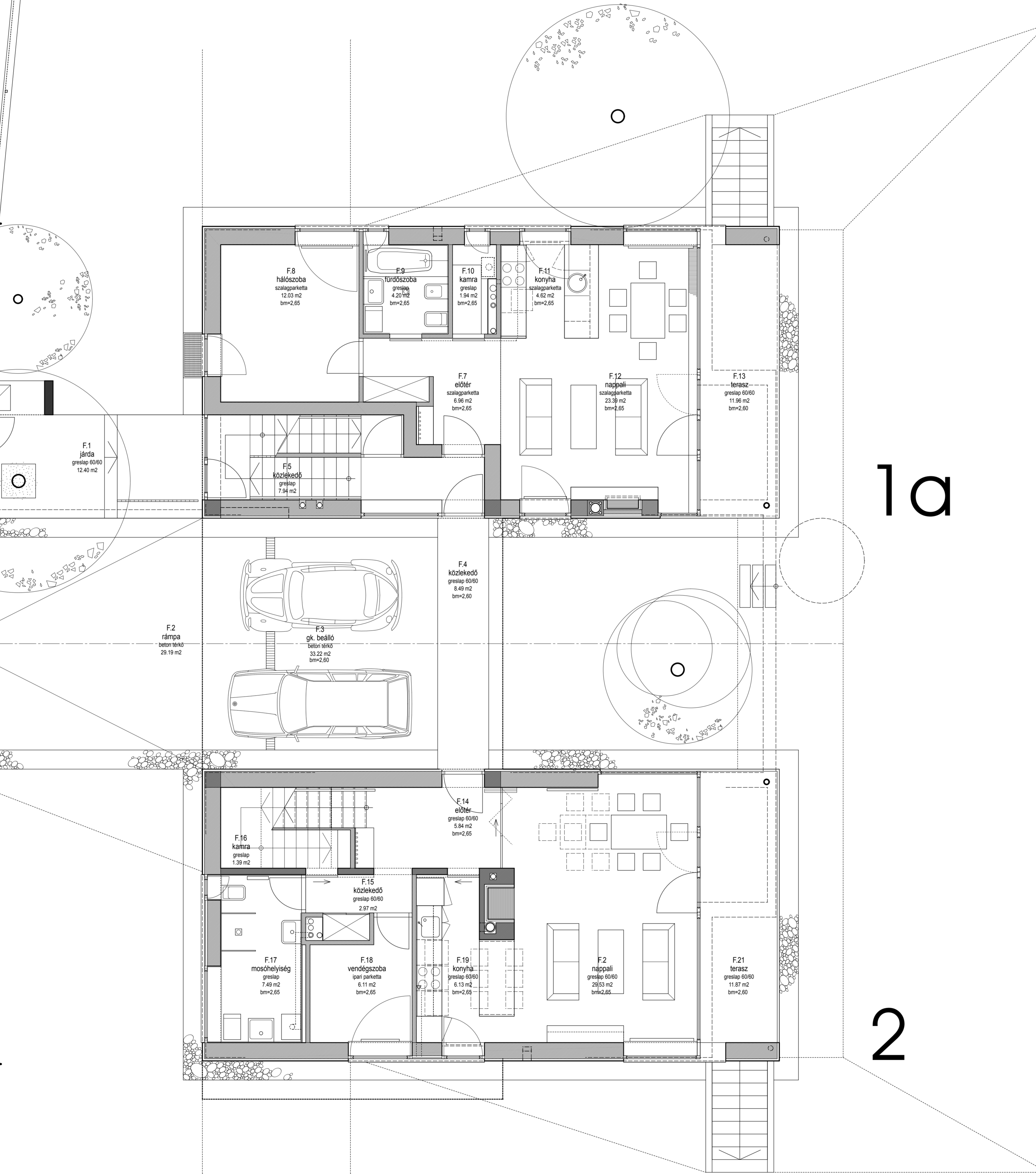
földszint alaprajz
