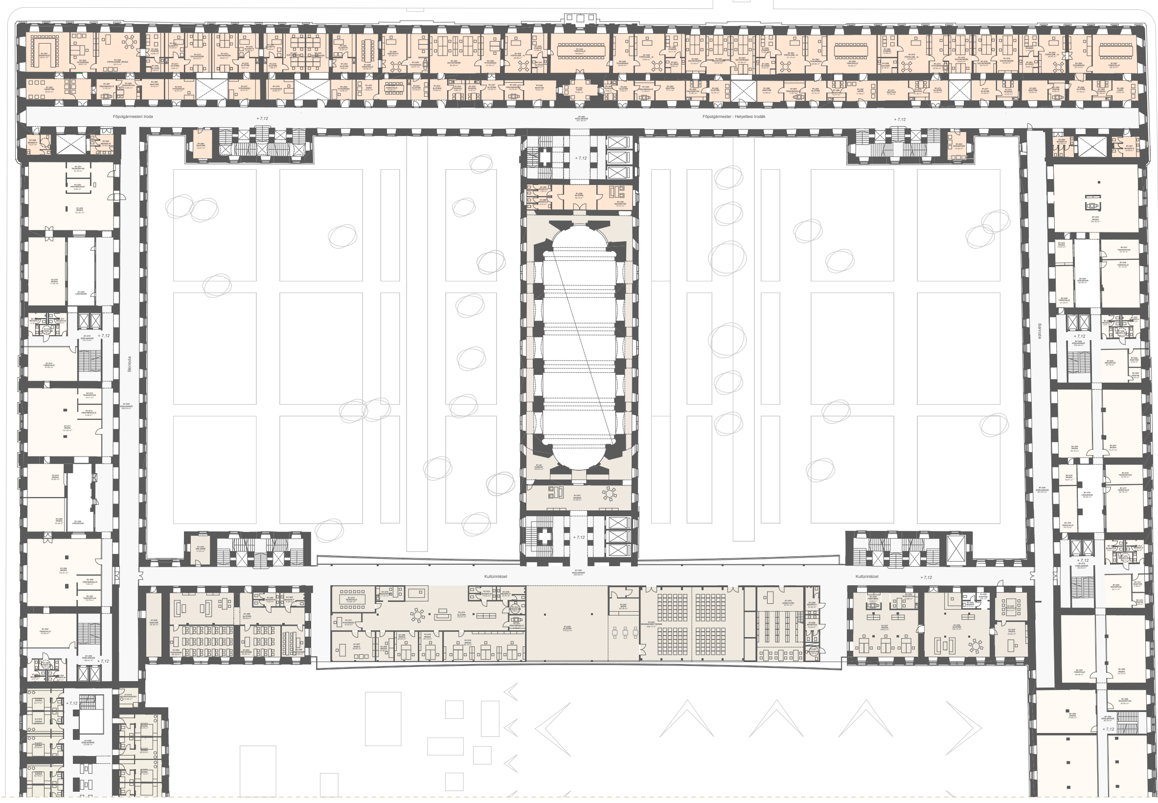
1. EMELETI ALAPRAJZ 2
