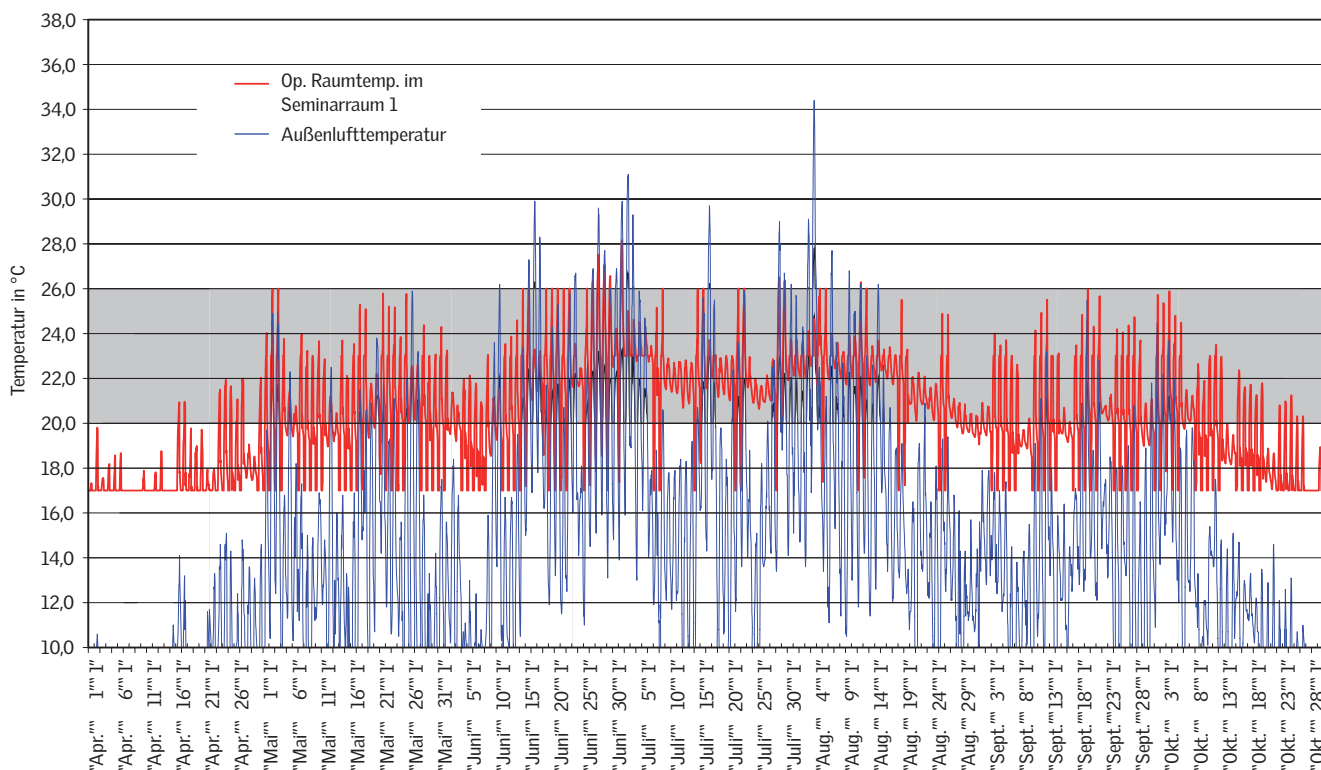
Sommerliche Raumtemperaturen
