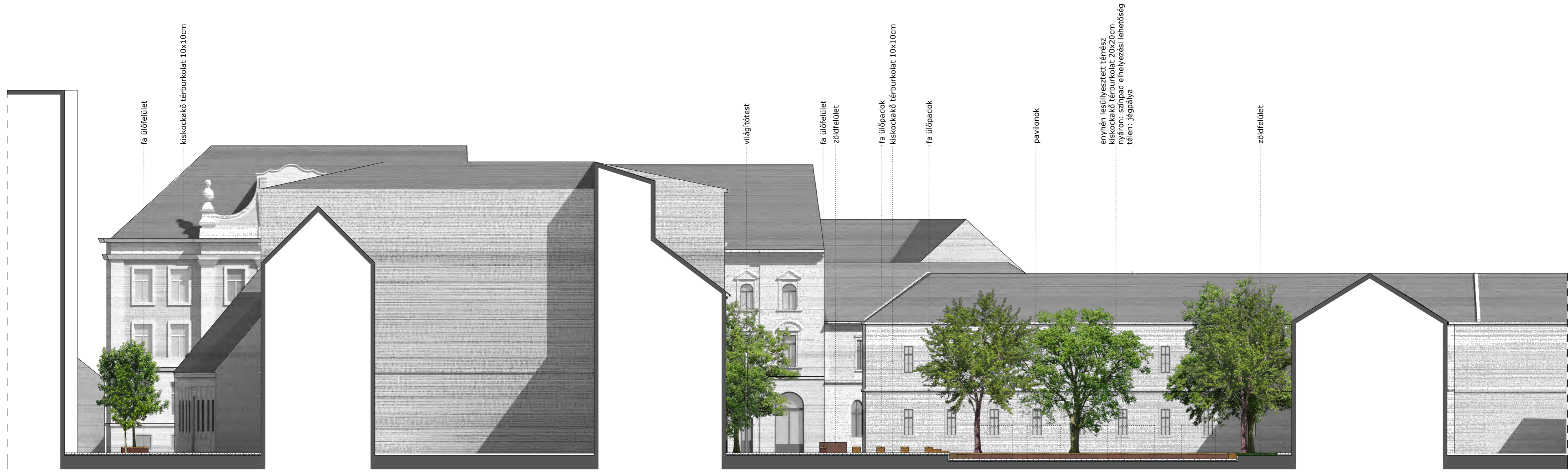
B-B metszet
