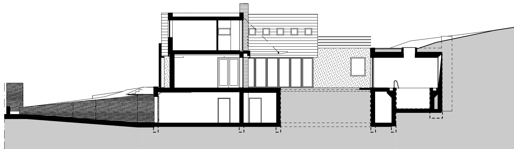
H2 Metszet
