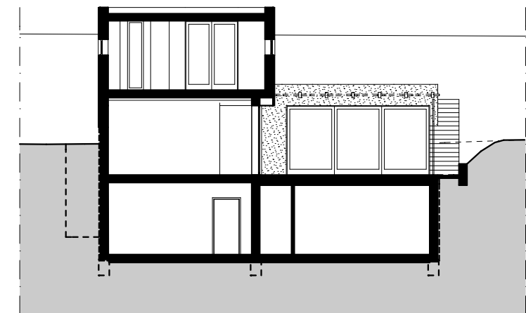
V2 Metszet
