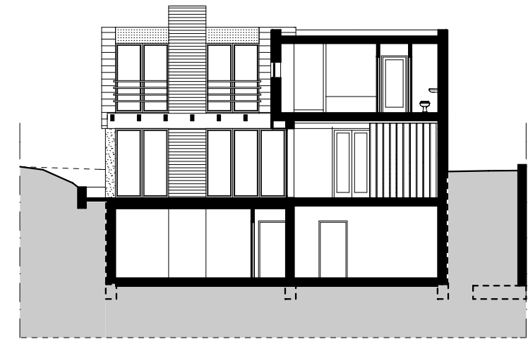
V1 Metszet
