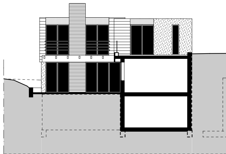
Keleti homlokzat
