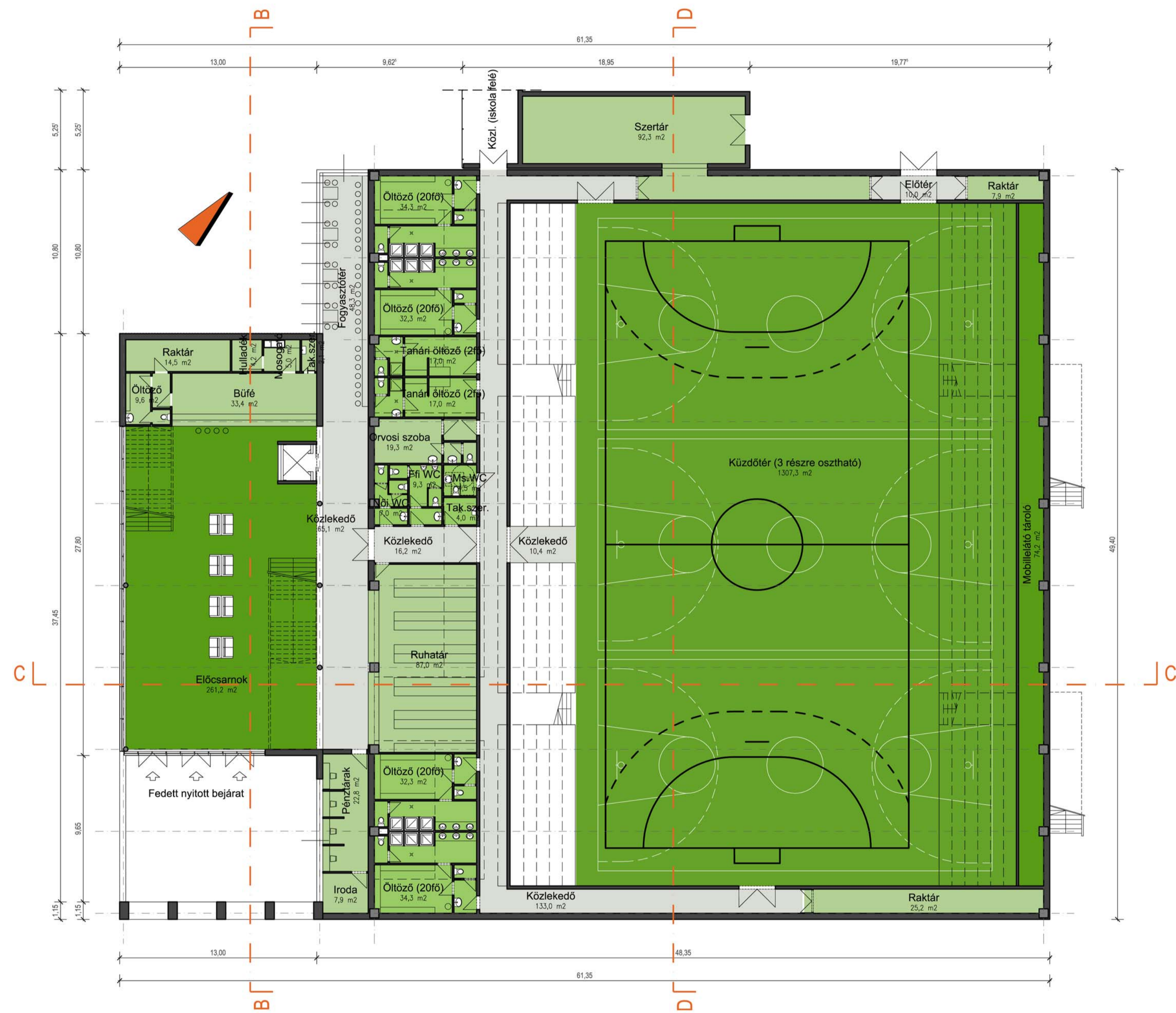
Földszinti alaprajz
