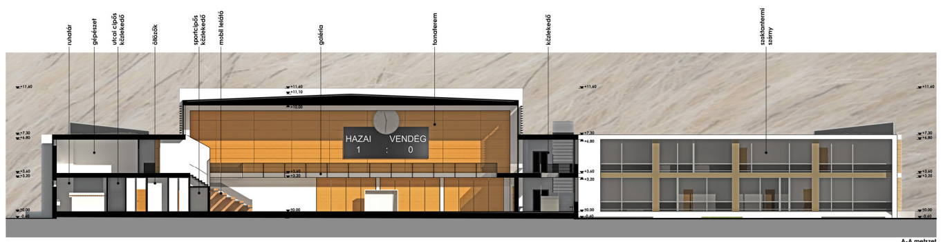
A-A metszet
