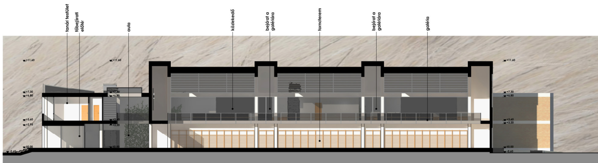
B-B metszet
